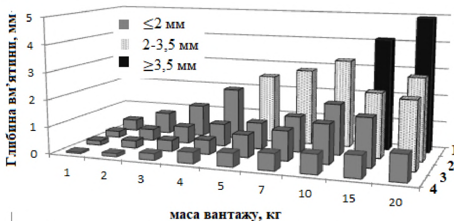
Рис. 1. Ударна стійкість бетонів через 28 днів тверднення
