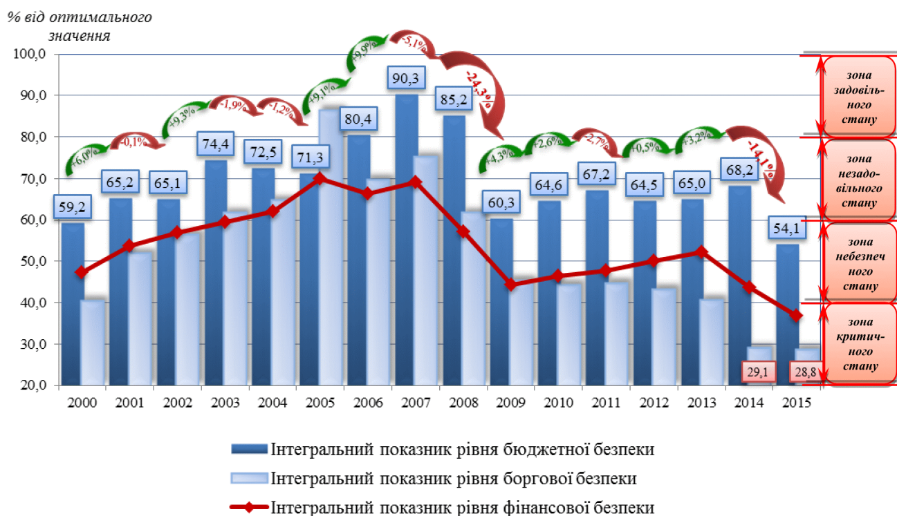
Рис. 1. Динаміка інтегрального індексу бюджетної безпеки України протягом 2000-2015 рр
