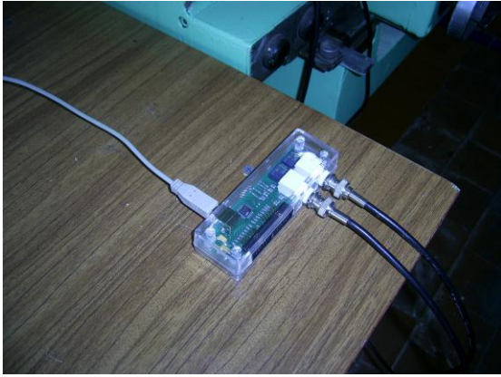
Рисунок 1 – Трикомпонентний динамометр
