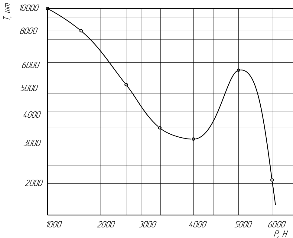
Рисунок 2 – Експериментальна залежність стійкості свердла від осьового зусилля
