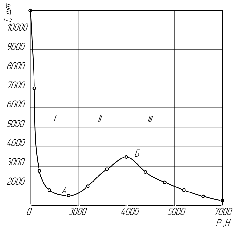
Рисунок 3 – Графік залежності стійкості свердла від осьового зусилля різання в лінійних координатах.
