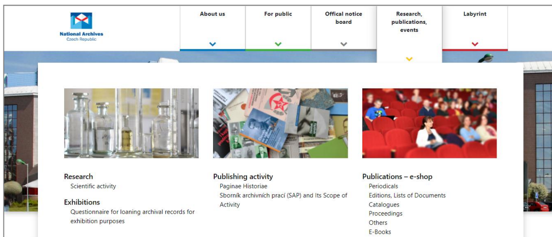
Рисунок 2.2.8 – Науково-інформаційний розділ [42]
