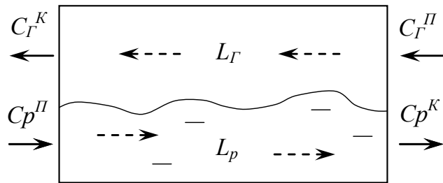
Рис.12.1. Схема абсорбера
