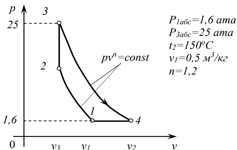
Рис. 4.12 Цикл в p - v координатах
