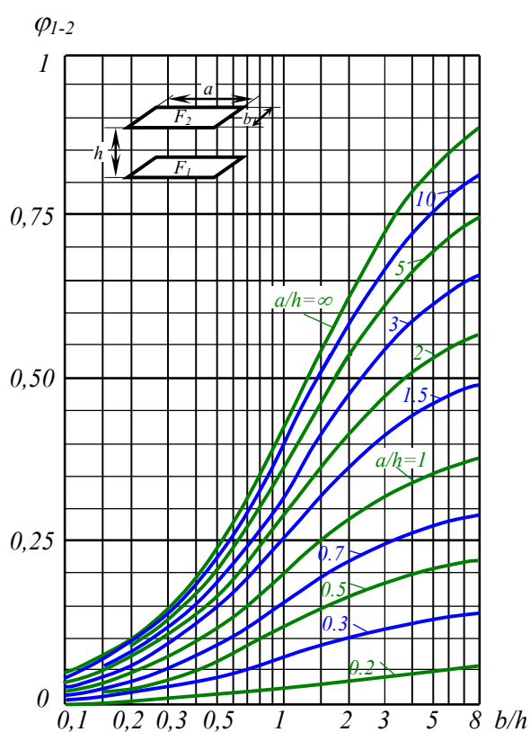
Рис. Г.1. Діаграма для визначення коефіцієнта опромінення для паралельно розташованих поверхонь
