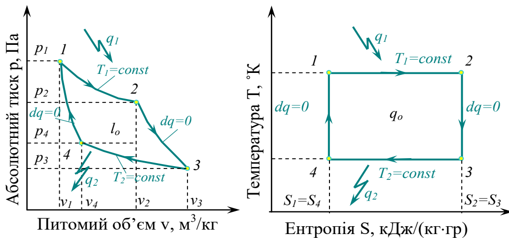
Рис. 3.5. Найпростіший цикл Карно в P-v і T-S – координатах [1]
