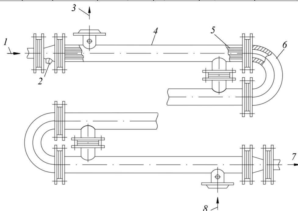
Рис. Е.1. Конструкція водо-водяного кожухотрубного теплообмінника ( за схемою протитечії):
