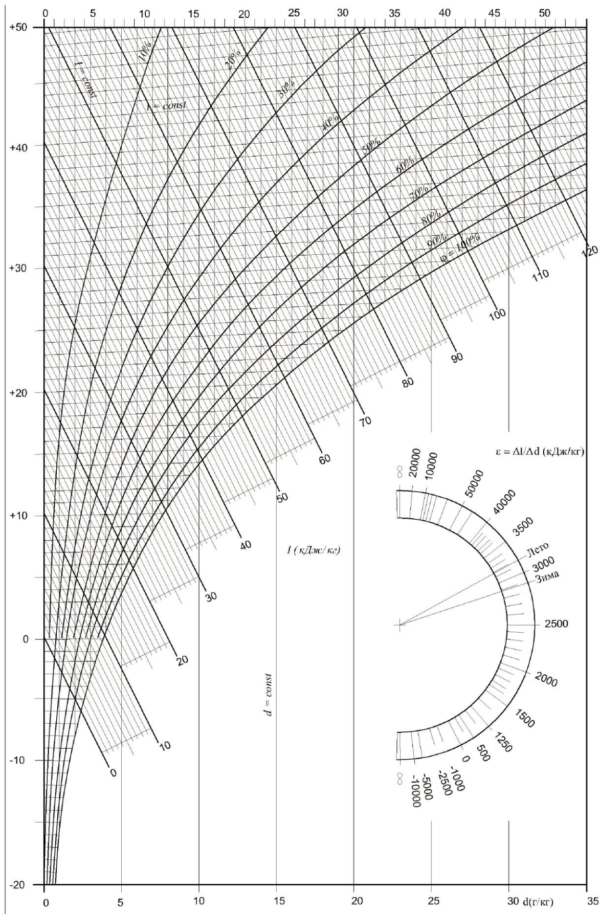
Рис. 5.1. I-d-діаграма вологого повітря
