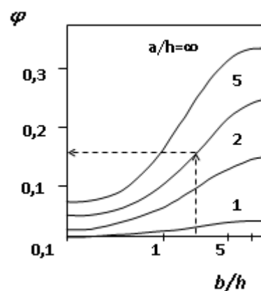
Рис. 8.4. Визначення коефіцієнта опромінення за діаграмою
