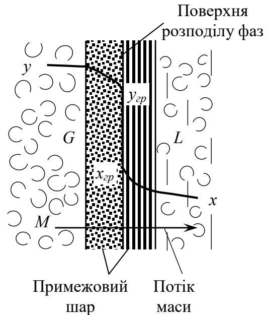
Рис.11.1. Схема процесу масопередавання
