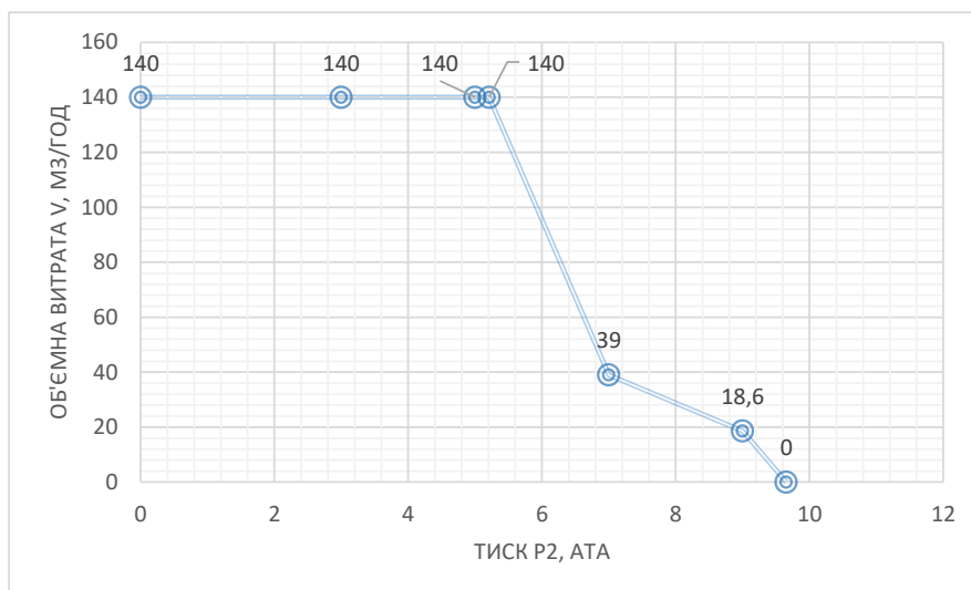
Графік залежності об'ємних витрат від тиску в зовнішньому середовищі
