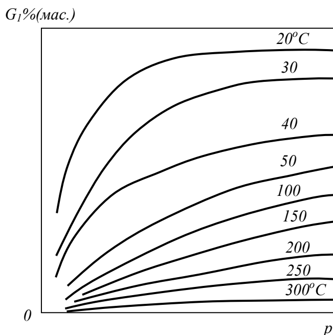
Рис. 12.5. Сітка ізотерм адсорбції
