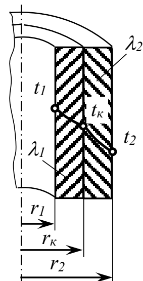
Рис. 7.4. Двохшарова циліндрична стінка
