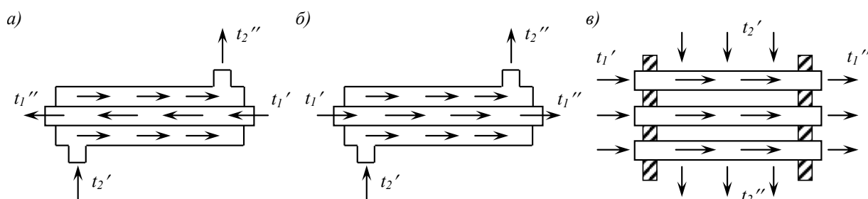
Рис.10.2. Напрямки руху теплоносіїв у теплообмінниках
