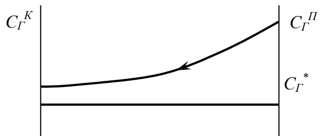
Рис.12.2. Концентрація газової фази в абсорбері
