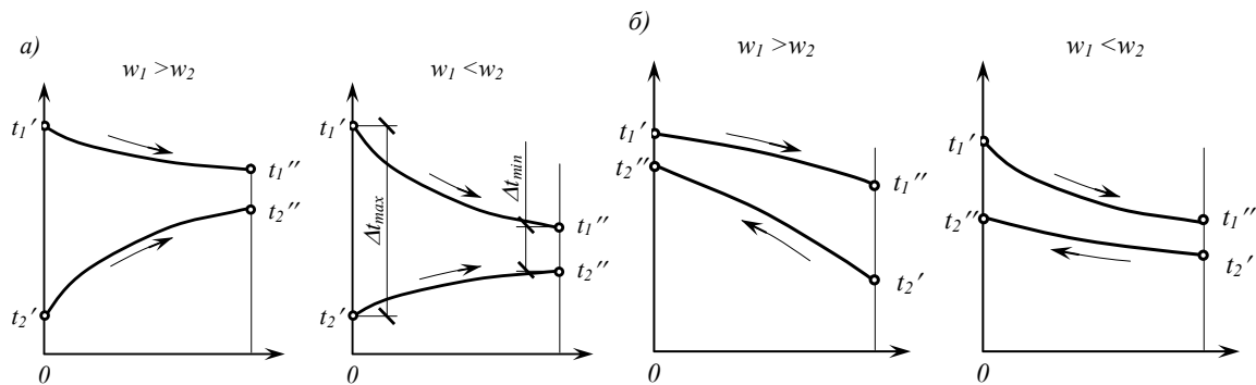
Рис. 10.3. Зміна температур теплоносіїв: а – прямоstrумінь; б – протиструмінь
