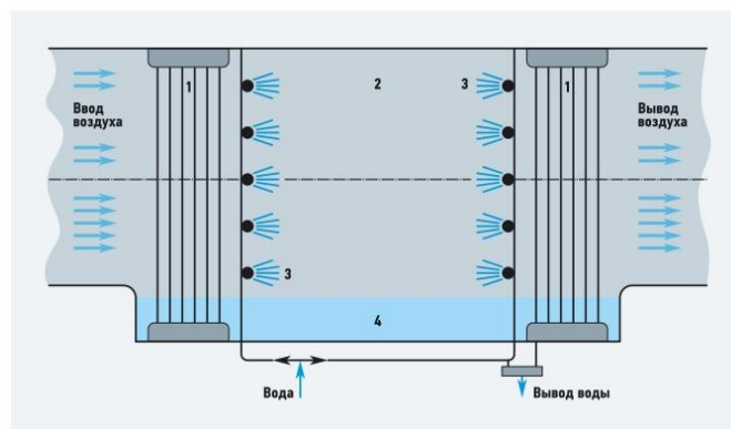
Рис. 3. Камера орошения (КО) [1 — наплеватель; 2 — корпус; 3 — форсунка; 4 — поддон]
