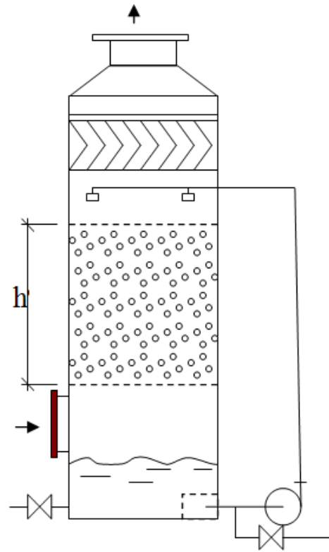
Рис.12.4. Абсорбер
