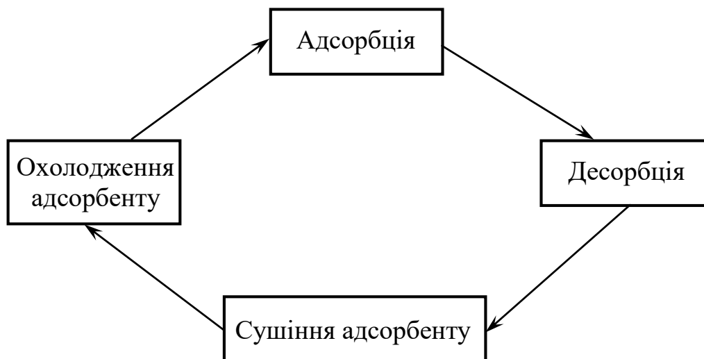
Рис.12.7. Принцип роботи адсорберів з нерухомим поглинальним шаром
