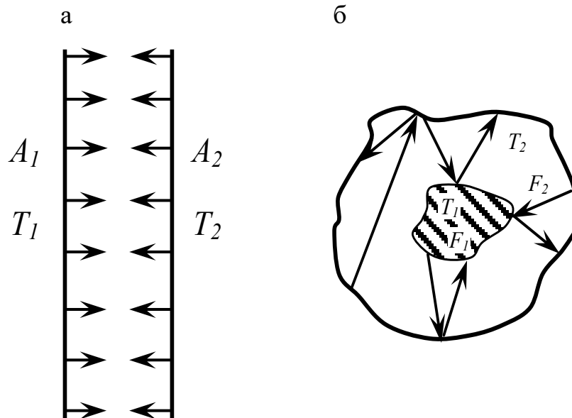
Рис. 8.5. Варіанти розташування теплообмінних поверхонь а – дві паралельні поверхні; б – поверхня 1, з усіх боків оточена поверхнею 2
