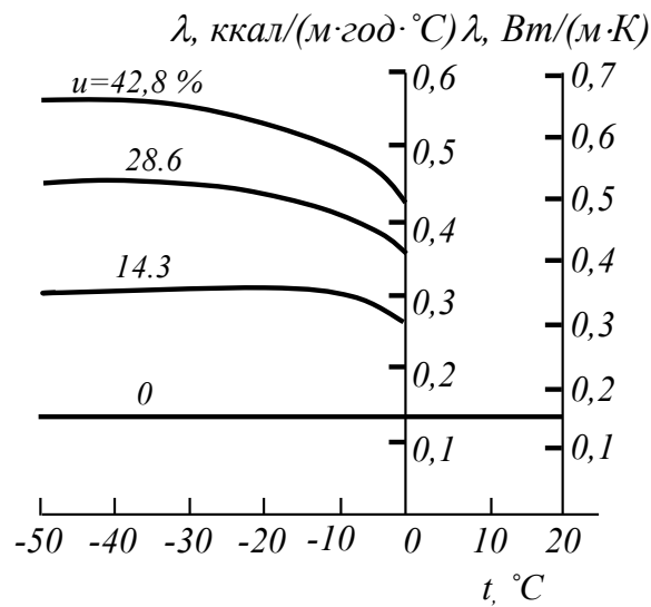
Рис.6.3. Теплопровідність вологого піносілікату при від'ємних температурах
