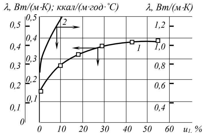
Рис. 6.2. Залежність теплопровідності матеріалу ( \lambda ) від його вологовмісту ( u ): 1– газосилікат, 2– червона цегла
