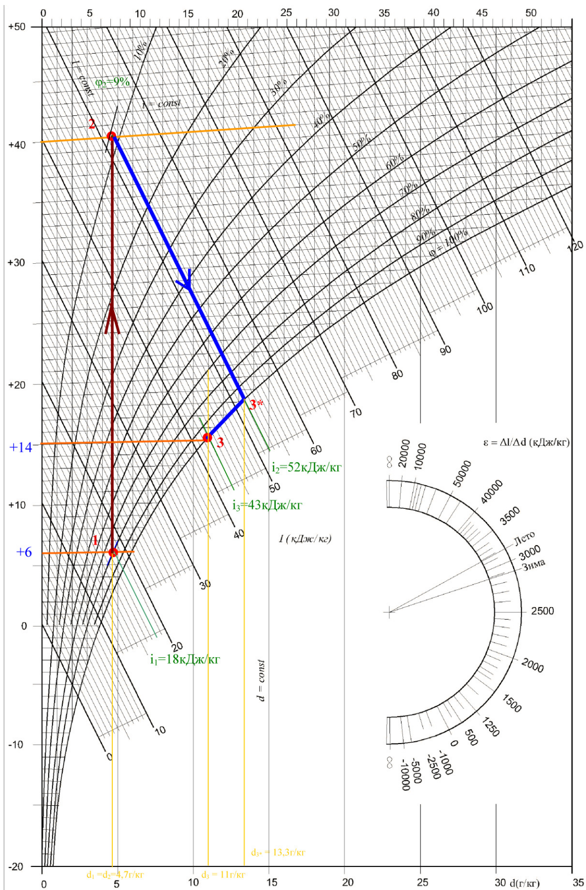
Рис. 5.4. I-d-діаграма вологого повітря
