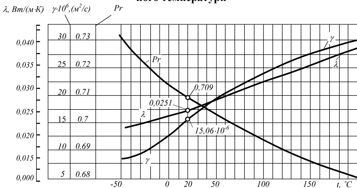
Рис. Д.1. Графік залежності \lambda , \gamma повітря від значення його температури
