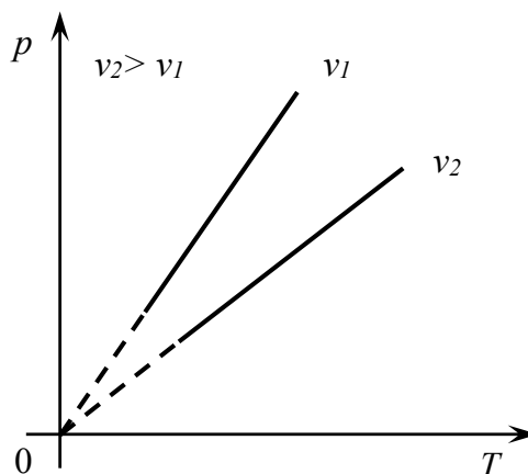
Рис. 1.3. Закон Шарля
