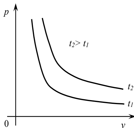
Рис. 1.1. Закон Бойля – Маріотта
