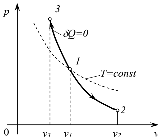
Рис. 3.4. Адіабатний процес
