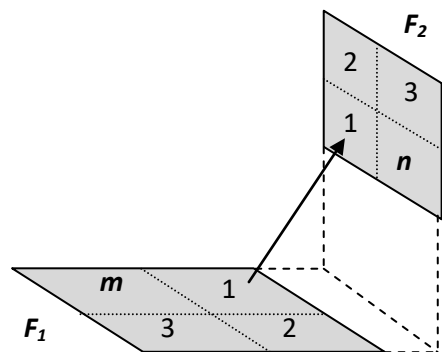
Рис. 8.3. Властивість розподіленості
