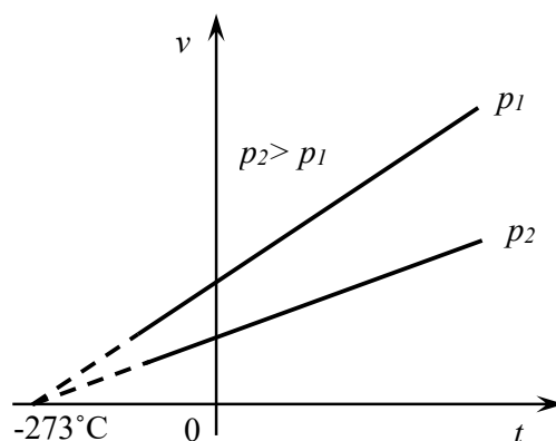
Рис. 1.2. Закон Гей-Люссака
