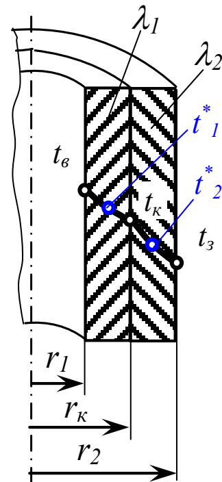
Рисунок 7.6– Побудова температурного поля багатошарової циліндричної стінки
