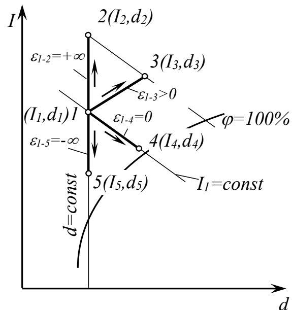
Рис. 5.2. Процеси на I-d-діаграмі
