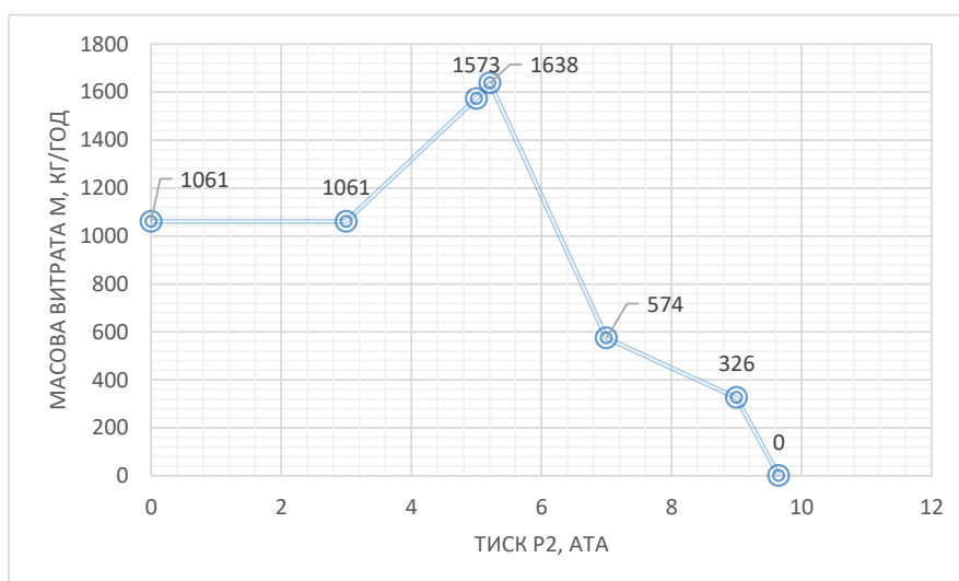
Графік залежності масових витрат від тиску в зовнішньому середовищі
