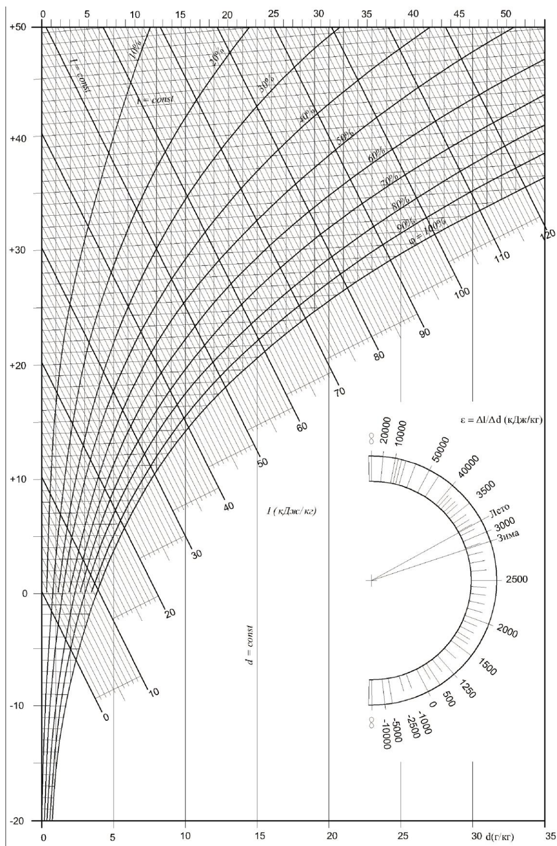
Рис. В.1. I-d-діаграма вологого повітря при 745 мм.рт.ст.
