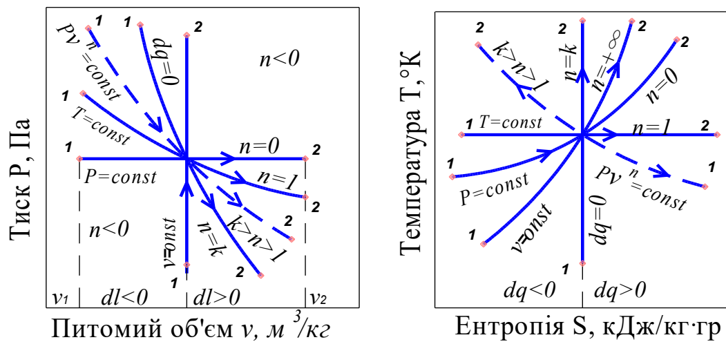
Рис. 3.6. Графіки процесів ідеального газу в координатах P–v та T–S [1]
