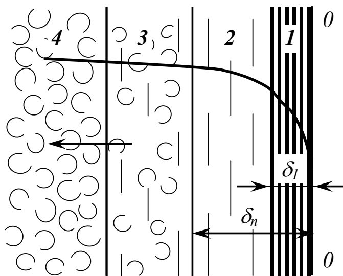
Рис. 11.2. Структура масообмінного потоку:
