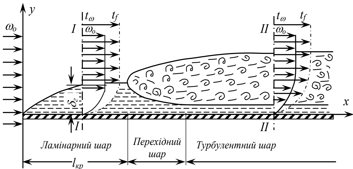
Рис. 9.1. Виникнення примежового шару при обтіканні тонкої пластини
