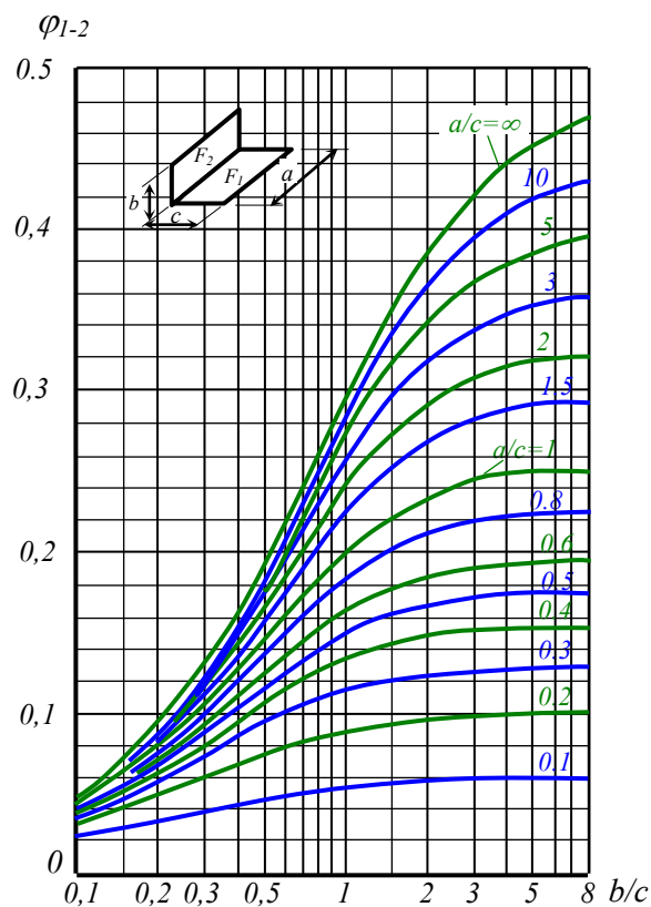
Рис. Г.1. Діаграма для визначення коефіцієнта опромінення для перпендикулярно розташованих поверхонь
