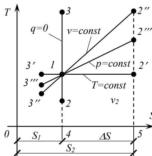
Рис. 3.3. Процеси в T-S координатах
