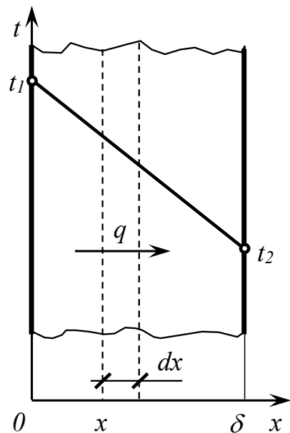
Рис. 7.1. Розподіл температур в одношаровій плоскій стінці
