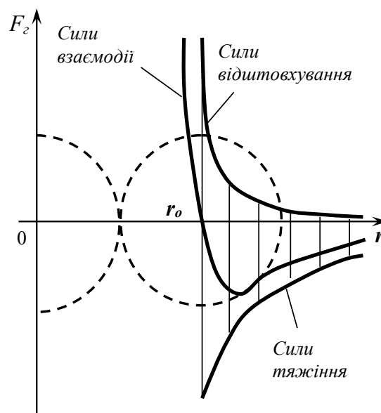
Рис. 2.1. Ван-дер-ваальсові сили
