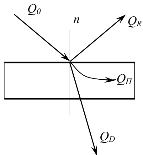
Рис. 8.1. Розподіл випромінювання
