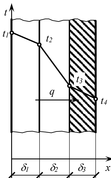
Рис. 7.2. Розподіл температур у багатошаровій плоскій стінці
