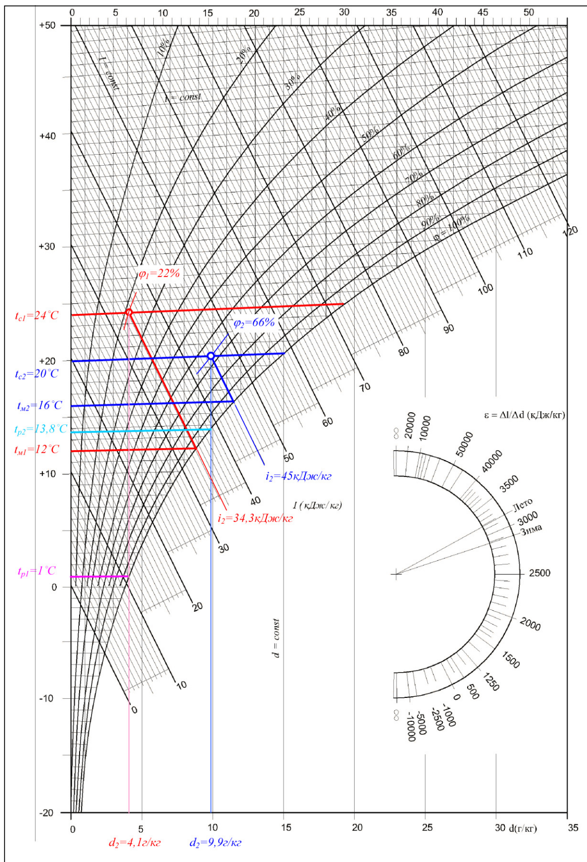
Рис. 5.3. Побудова точок на I-d-діаграмі
