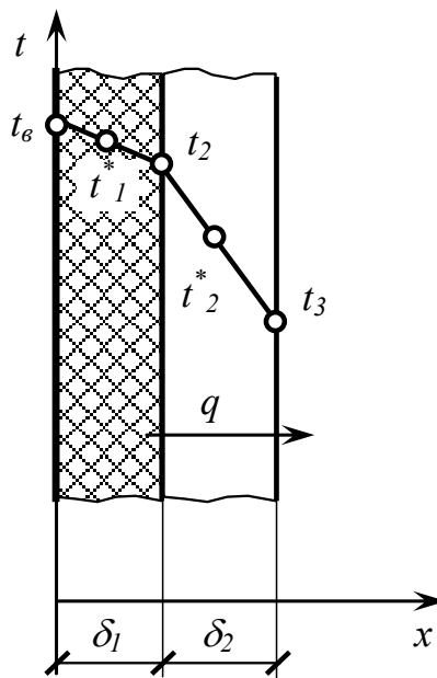
Рис. 7.5. Побудова температурного поля багат шарової плоскої стінки
