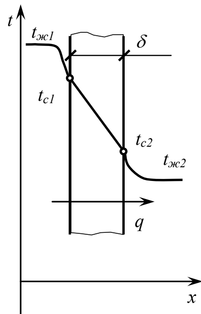
Рис.10.1. Теплопередавання через плоску стінку
