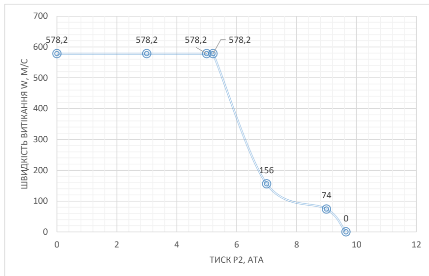
Графік залежності швидкості витікання від тиску в зовнішньому середовищі
