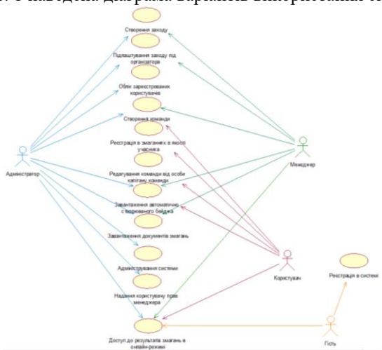
Рис.1.Діаграма прецедентів (Use Case Diagram)
