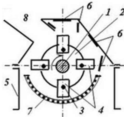
Рис. 1. Основні конструктивні елементи молоткової дробарки:
