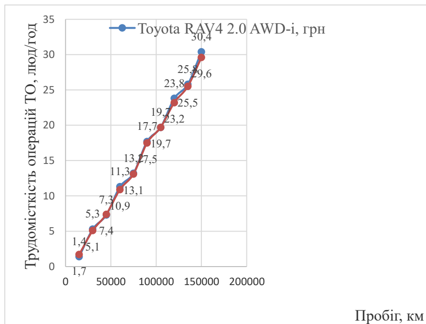
Рис. 2. Залежності трудомісткостей ТО за пробігом в кожні 15000 км кросоверів Toyota RAV4 2.0 AWD-i та Toyota RAV4 Hybrid AWD-i
