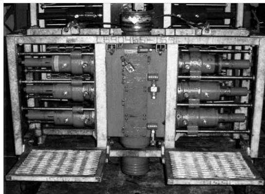
Рис. 3. Привентор (WCV)
