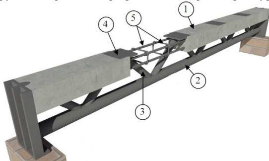
Рис. 7. Загальний вигляд зразка серії Б-3, 1. залізобетонна лінійна складова; 2,3 труби; 4. анкери; 5 арматурна сітка.
