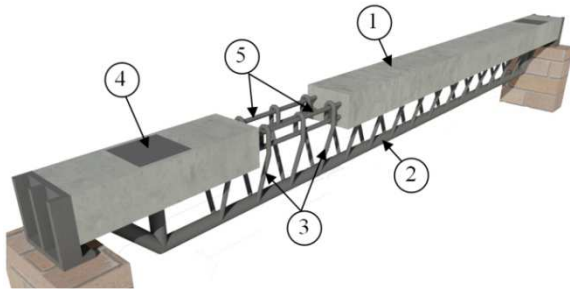
Рис. 5. Загальний вигляд зразка серії Б-1, 1. залізобетонна лінійна складова; 2. дротяна арматура; 3,4. анкери; 5. арматурна сітка.
