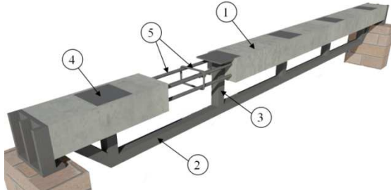
Рис. 6. Загальний вигляд зразка серії Б-2, 1. залізобетонна лінійна складова; 2,3 труби квадратного профілю; 4. анкери; 5 арматурна сітка.
