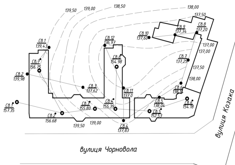
Рисунок 3 – Карта поверхні водотривкого шару на майданчику по вул. Чорновола, 2б:
