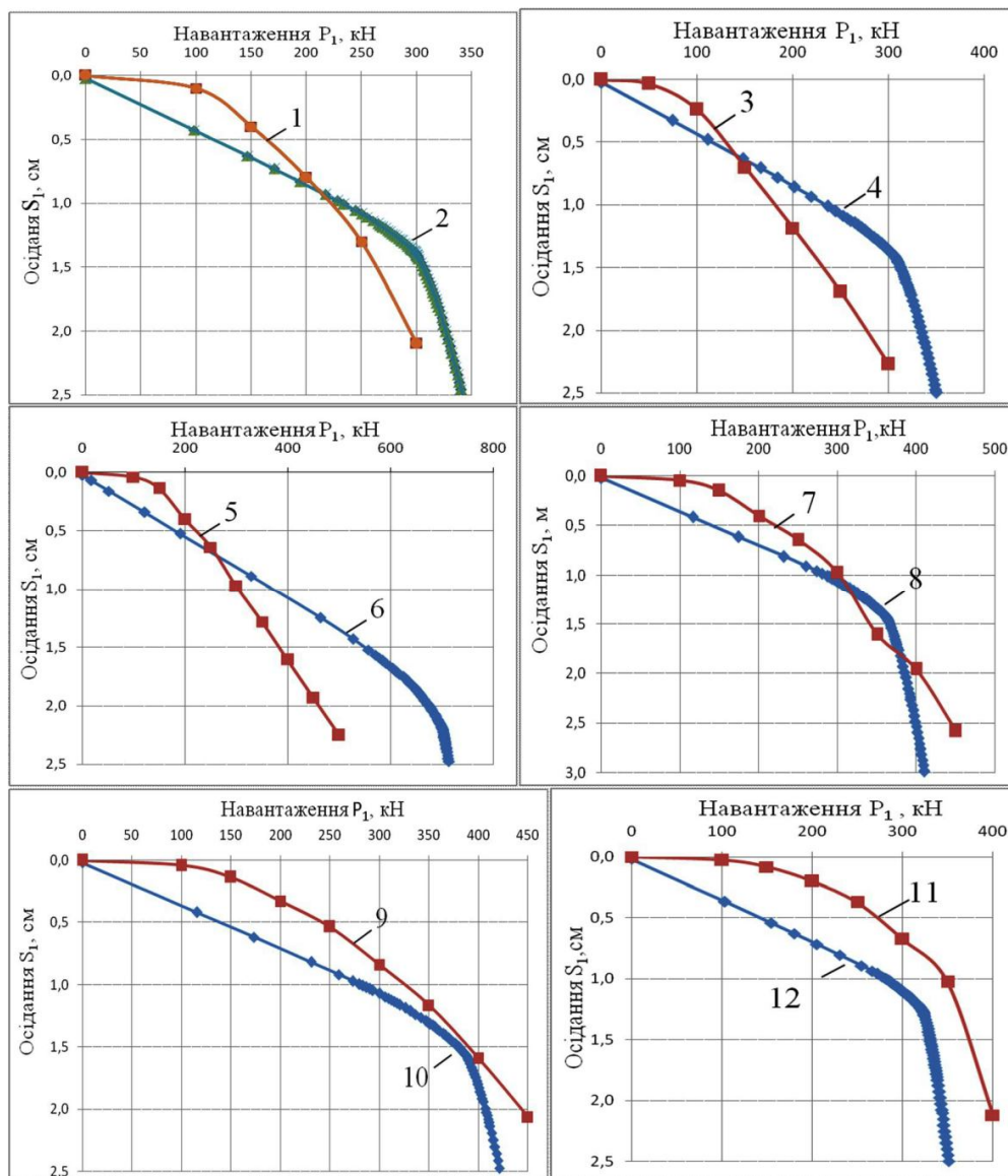
Рисунок 4 – Результати статичного випробування паль та моделювання за допомогою програмного комплексу PLAXIS: графіки 1, 3 – палі С 7-35; графік 5 – палі С 14-35; графіки 7, 9, 11 – палі С 9-30 за результатами статичного випробування; графіки 2, 4 – палі С 7-35; графік 6 – палі С 14-35; графіки 8, 10, 12 – палі С 9-30 за результатами моделювання у програмному комплексі PLAXIS
