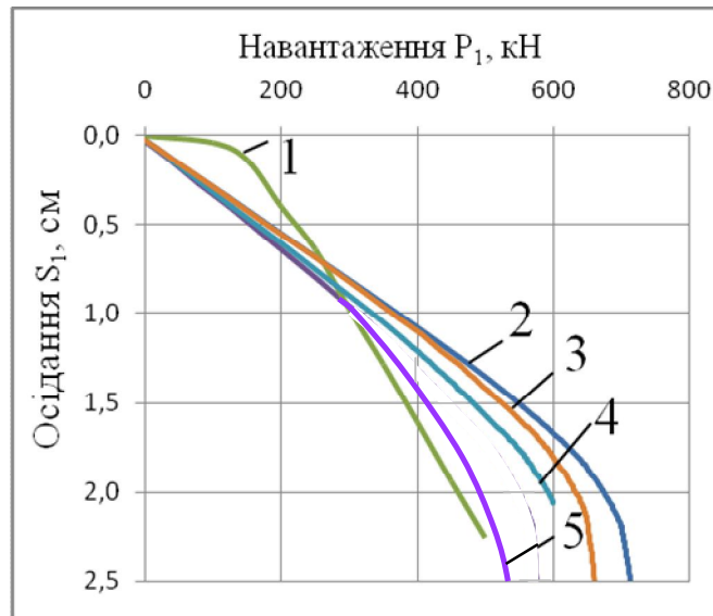
Рисунок 5 – Порівняння графіка залежності осідання палі С 14-35 від навантаження за результатами статичного випробування та за результатами моделювання в програмному комплексі PLAXIS з різними характеристиками ІГЕ-5:
