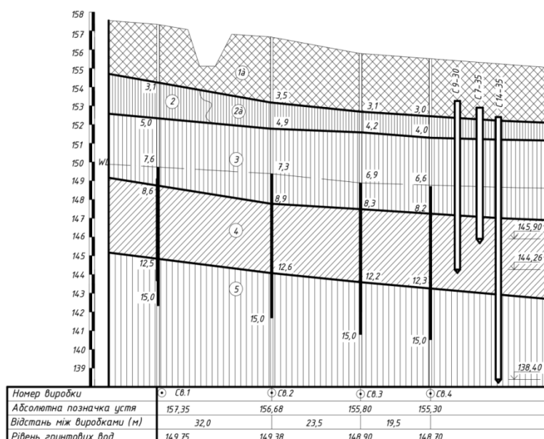
Рисунок 2 – Інженерно-геологічний розріз по вул. Чорновола, 2б
