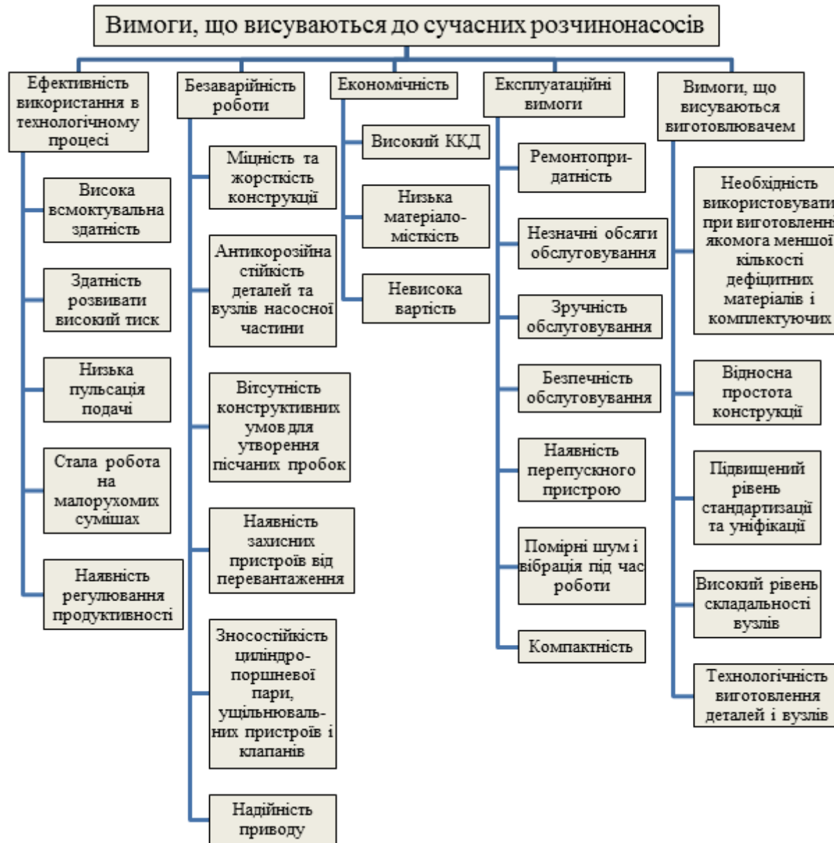
Рисунок 2 – Пропоновані до розчинонасосів вимоги
