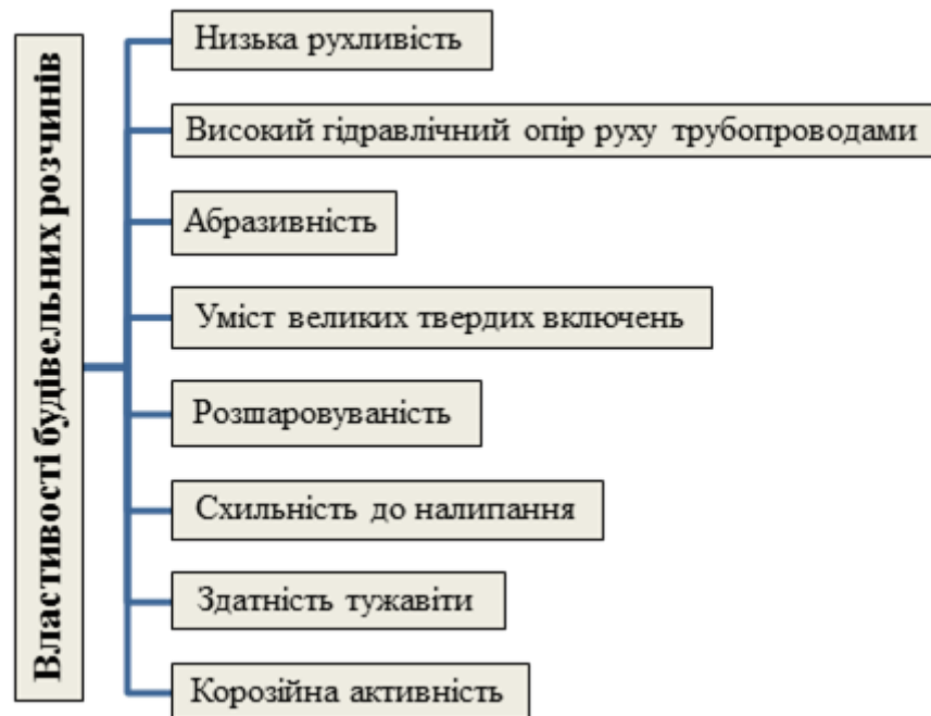
Рисунок 1 – Особливості будівельних розчинів, що ускладнюють роботу розчинонасосів
