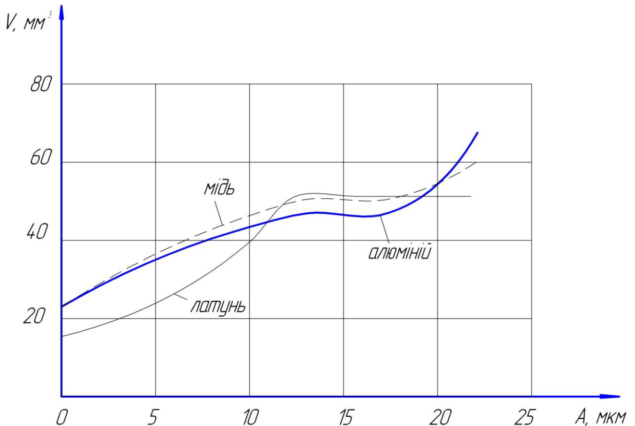
Рисунок 2 – Графіки залежності об'єму зшліфованого матеріалу V , мм 3 , від амплітуди коливань A , мкм
