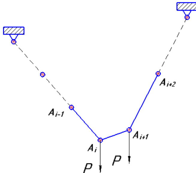
Рисунок 3. Дискретна модель розтягнутої нитки у формі параболи другого порядку.
