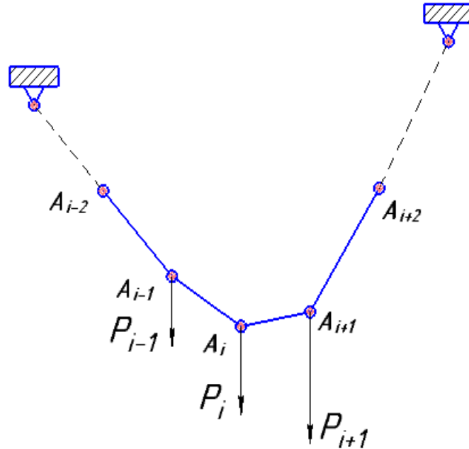
Рисунок 4. Дискретна модель розтягнутої нитки у формі параболі третього порядку.
