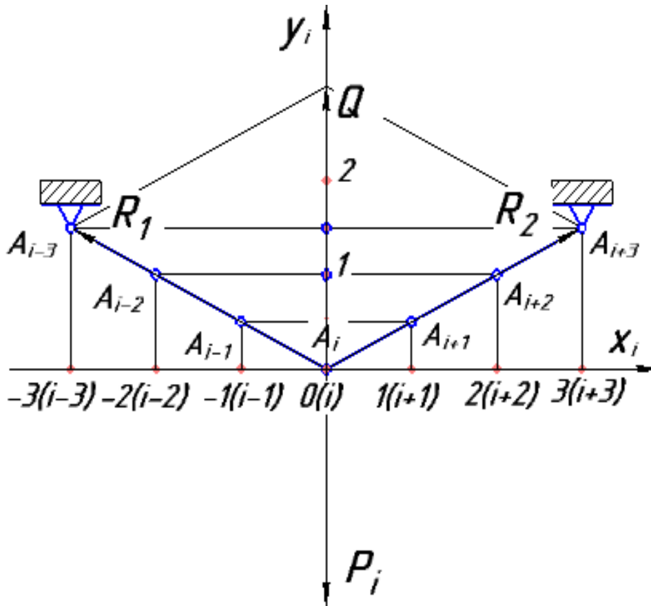
Рисунок 2. Дискретна модель прямих y = -0,5x та y = 0,5x у формі нерозтяжної натягнутої нитки
