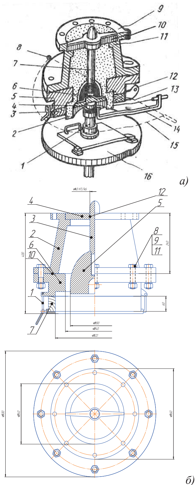
Рисунок 2 – Пресова головка: а) 3-D зображення з'єднання зі столом; б) складальне креслення
