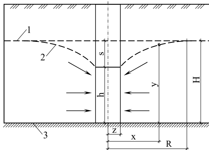
Рис. 3.11. Розрахункова схема припливу води до досконалого колодязя в ненапірному водоносному шарі: 1 – рівень ґрунтової води; 2 – лінія депресії; 3 – водотривкий шар
