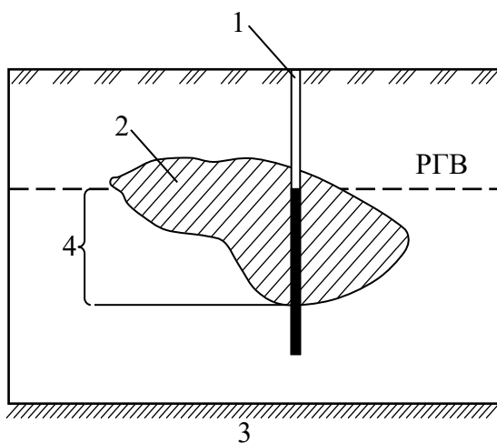
Рис. 3.5. Утворення місцевого напору в ґрунтових водах: 1 – свердловина; 2 – місцевий водотривкий шар; 3 – водотривкий шар масиву; 4 – місцевий напір
