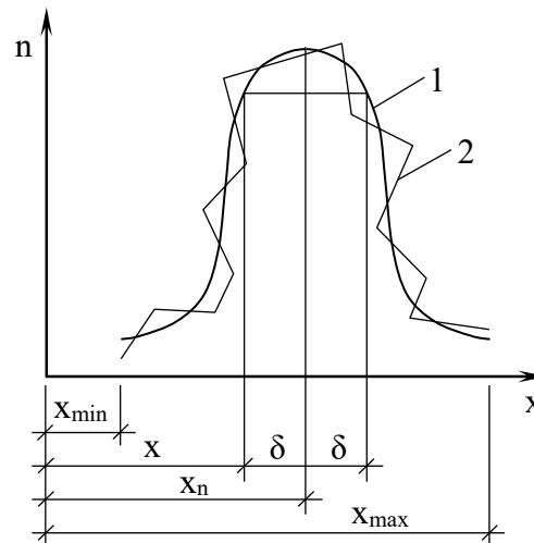
Рис. 4.19. Статистичні криві розподілу значень фізико-механічних параметрів: 1 – теоретична; 2 – дослідна
