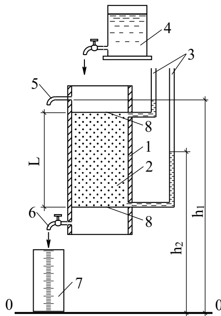
Рис. 3.8. Схема приладу Дарсі: 1 – робочий циліндр; 2 – пісок; 3 – п'єзометричні трубки; 4 – бачок із водою; 5 – зливна трубка; 6 – зливний кран; 7 – мірний посуд; 8 – сітка
