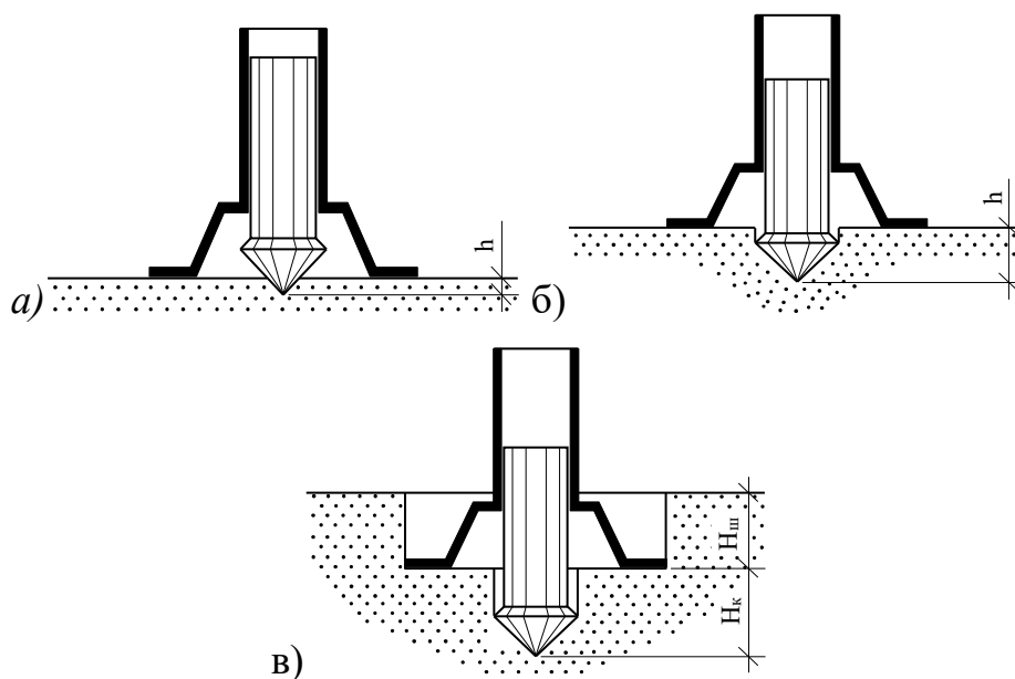
Рис. 4.16. Схема випробування ґрунтоміром-пенетрометром Л-13 різних ґрунтів: а – пористі та пінисті тверді; б – пухкі зв’язні та ущільнені незв’язні; в – пухкі незв’язні та пилуваті
