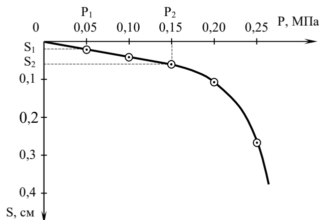
Рис. 5.12. Графік залежності осідання штампa від тиску
