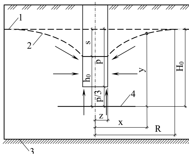
Рис. 3.12. Розрахункова схема припливу води до недосконалого колодязя в ненапірному водоносному шарі: 1 – рівень ґрунтової води; 2 – лінія депресії; 3 – водотривкий шар; 4 – умовний водотрив; s – динамічний рівень води; p – глибина води в колодязі
