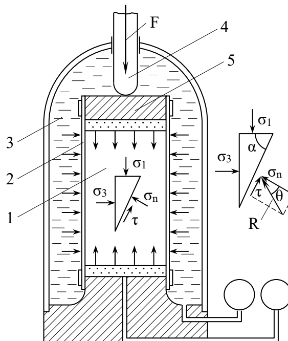
Рис. 4.8. Схеми приладу трьохосового стиснення (стабілометра) (а) та напруженого стану зразка ґрунту в ньому (б)
