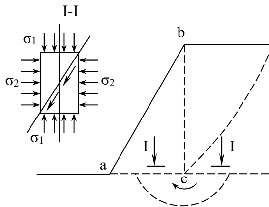
Рис. 2.31. Схема напруженого стану на схилі
