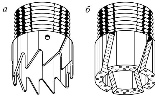
Рис. 5.6. Види бурових коронок
