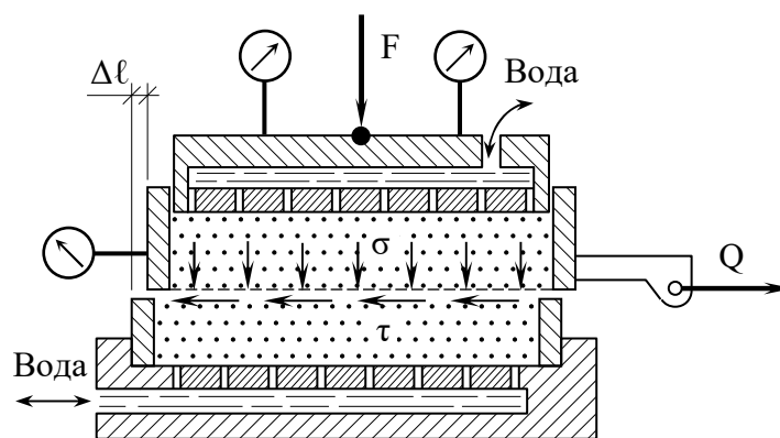
Рис. 4.10. Схема приладу для випробувань ґрунтів на пряме зрушення
