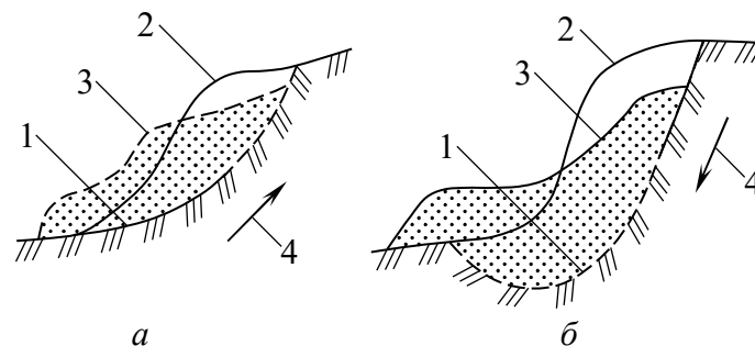
Рис. 2.32. Класифікація зсувів за А.П. Павловим: а – деляпсивний; б – детрузивний; 1 – підосва зсуву; 2 – схил до зсуву; 3 – схил після зсуву; 4 – напрямок утворення поверхні ковзання
