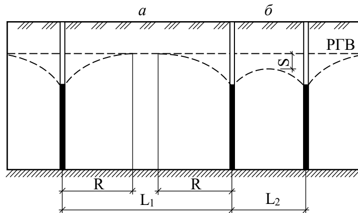
Рис. 3.15. Схема взаємного розташування свердловин: а – взаємодії немає; б – взаємодія є; S – величина зниження рівня води; R – радіус депресії; L_1, L_2 – відстані між свердловинами
