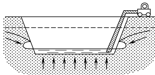
Рис. 2.26. Суфозія при відкритому водовідливі: 1 – рівень ґрунтової води; 2 – ніша; 3 – зона послаблення основи
