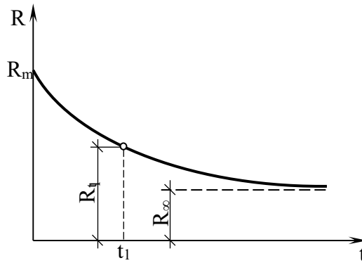
Рис. 4.23. Крива тривалої міцності ґрунту
