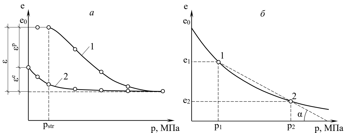
Рис. 4.5. Компресійні криві: а – загальний вигляд (1 – навантаження; 2 – розвантаження); б – розрахункова схема для визначення коефіцієнта відносної стисливості
