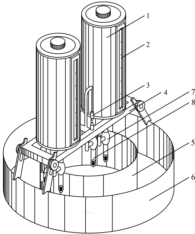
Рис. 3.19. Прилад для визначення водопроникності ґрунтів: 1 – бачок; 2 – водомірна шкала; 3 – висок; 4 – штатив; 5 – внутрішнє кільце; 6 – зовнішнє кільце; 7 – повітряна трубка 8 – водоспускна трубка
