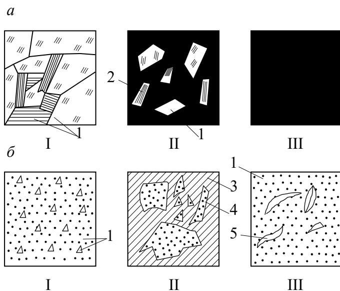
Рис. 1.1. Види структур гірських порід: а – магматичні породи, I – повнокристалічна, II – напівкристалічна; III – аморфна; б – осадові породи, I – уламкова (псамітова); II – брекчієвидна; III – органогенна (фітопелітова), 1 – зерна, 2 – аморфна речовина; 3 – глина, 4 – уламки; 5 – залишки рослин
