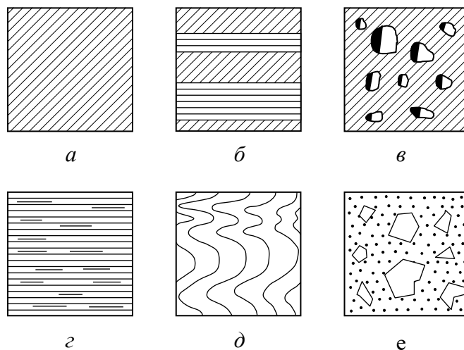
Рис. 1.2. Текстура гірських порід: а – масивна; б – шарувата; в – макропориста; з – розсіяна; д – флюїдальна, е – хаотична
