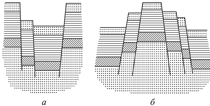
Рис. 2.2. Дислокації, що виникають під час розривних рухів земної кори: а – грабен; б – горст
