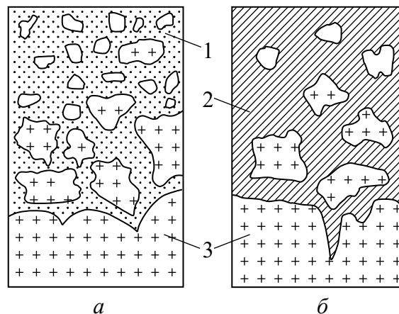
Рис. 2.6. Елювій при вивітрюванні: а – фізичному; б – хімічному; 1 – пісок; 2 – глина; 3 – корінна порода
