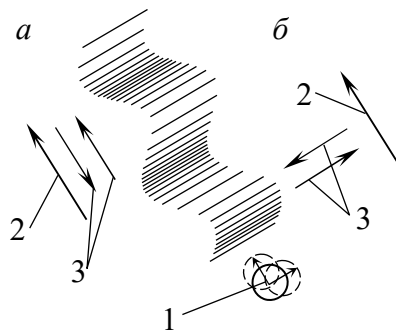
Рис. 2.4. Схема утворення сейсмічних хвиль: а – поздовжніх; б – поперечних; 1 – осередок землетрусу; 2 – напрям поширення хвилі; 3 – напрям коливання частинок
