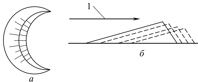
Рис. 2.15. Бархани: а – план; б – розріз; 1 – напрям вітру
