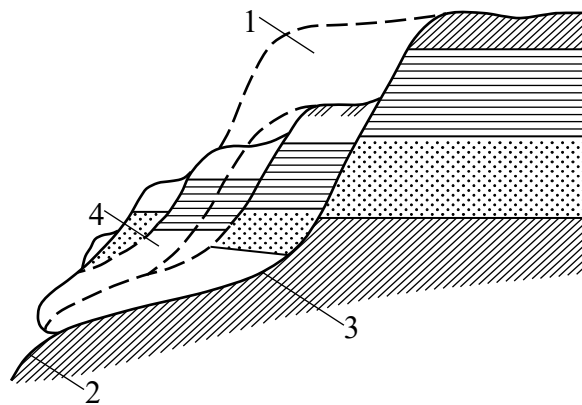
Рис. 2.30. Загальний вигляд зсуву: 1 – зсувний цирк; 2 – підшовка зсуву; 3 – поверхня ковзання; 4 – тіло зсуву
