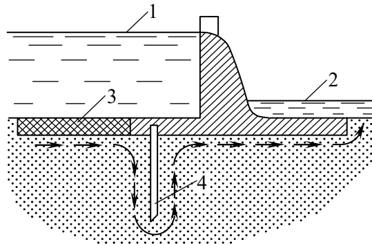
Рис. 2.25. Водозливна бетонна гребля на піщаній основі: 1 – верхній рівень води; 2 – нижній рівень води; 3 – понур; 4 – шпунтова стінка
