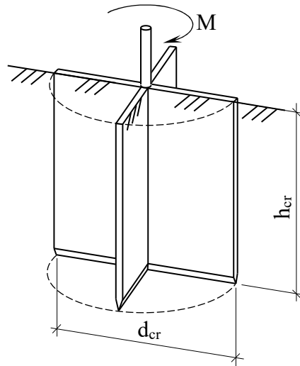
Рис. 4.17. Схема випробування ґрунтів методом обертального зрізу
