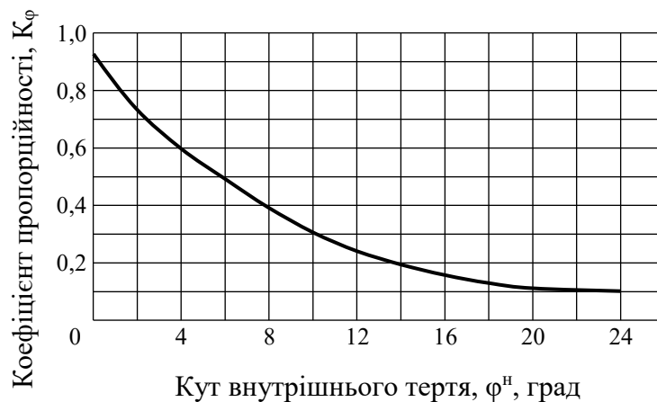
Рис. 4.18. Графік для визначення кута внутрішнього тертя за коефіцієнтом пропорційності K_{\varphi}
