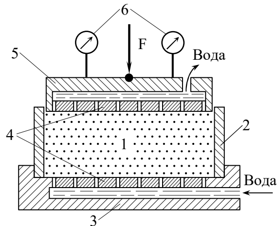
Рис. 4.4. Схема одометра для компресійних випробувань ґрунтів: 1 – зразок ґрунту; 2 – металеве кільце; 3 – дніще; 4 – тонкі отвори; 5 – штамп; 6 – індикатори годинникового типу
