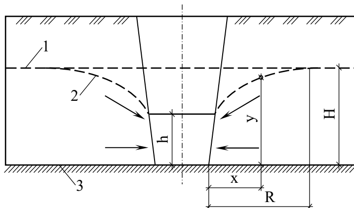
Рис. 3.14. Розрахункова схема припливу води до каналу: 1 – рівень ґрунтової води; 2 – лінія депресії; 3 – водотривкий шар
