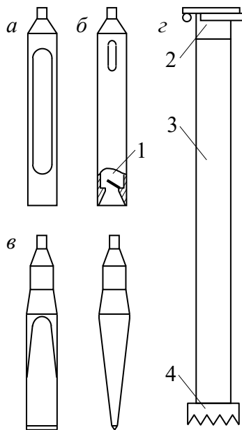
Рис. 5.4. Інструмент для ударно-канатного буріння: а – забивний стакан; б – желонка; в – долото; г – обсадна труба; 1 – клапан; 2 – наголовник; 3 – ланка обсадної труби; 4 – фреза
