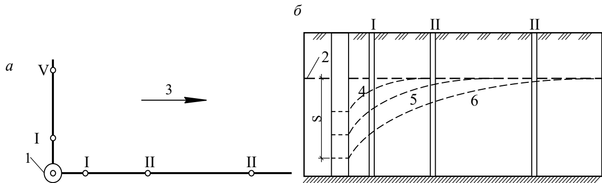
Рис. 3.17. Схема проведення дослідних відкачувань води: а – розташування свердловин; б – розріз за свердловинами I, II, III; 1 – центральна свердловина; 2 – рівень ґрунтових вод; 3 – напрям руху вод; 4, 5, 6 – лінії депресії при послідовних зниженнях рівня води
