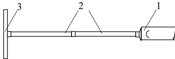
Рис. 5.2. Знаряддя для проведення ручного буріння: 1 – стакан; 2 – штанги; 3 – рукоятка
