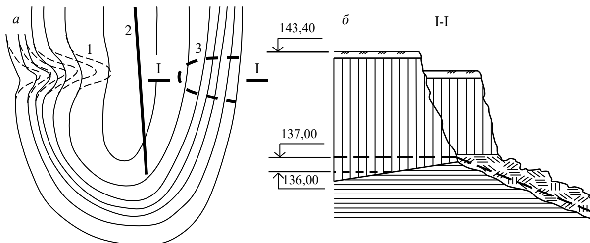
Рис.2.35. Схеми розвитку зсуву в районі с. Червоний Шлях: а – план; б – розріз по I-I; 1 – яр розвантаження ґрунтових вод; 2 – водогін; 3 – межі розвитку зсуву
