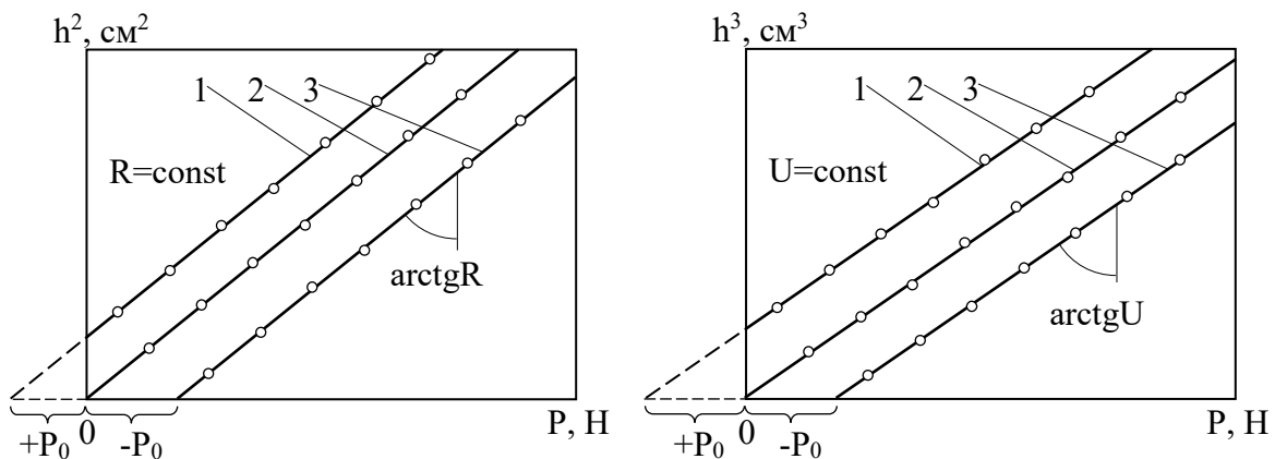
Рис. 4.15. Графіки penetраційних випробувань: а – зв'язного ґрунту; б – сипучого ґрунту
