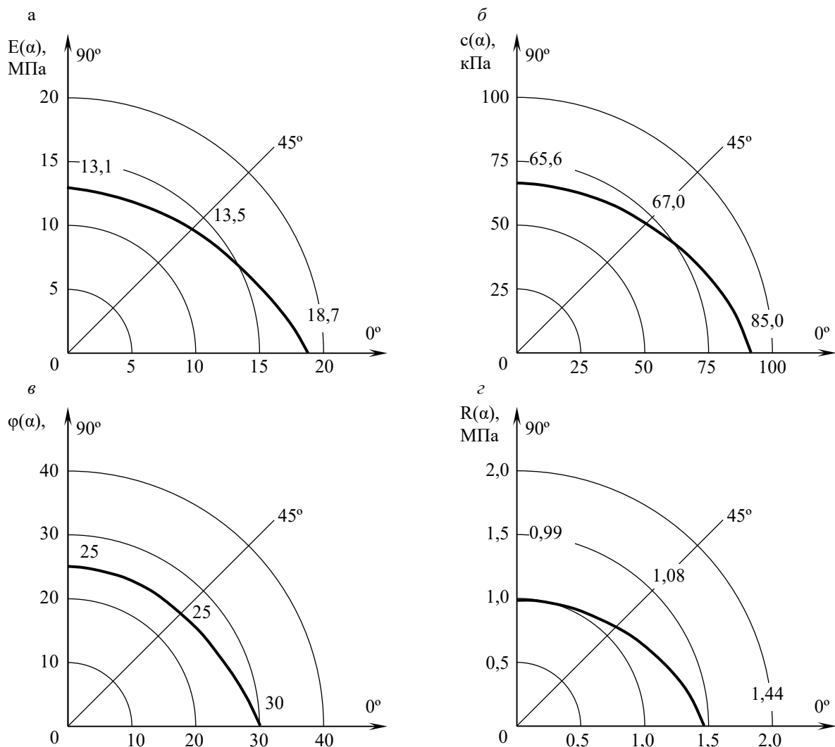
Рис. 4.21. Приклади годографів механічних характеристик лесового суглинка в характерній точці ущільненого шару ґрунтової подушки (за даними Ю.Л. Винникова): а – модуль деформації; б – питоме зчеплення; в – кут внутрішнього тертя; з – питомий опір penetрації
