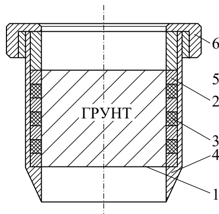
Рис. 4.7. Кільце для компресійних випробувань ґрунтів НУ «Полтавська політехніка імені Юрія Кондратюка»: 1 – кільце; 2 – металеві кільця; 3 – еластичні прокладки; 4 – циліндрична гільза з ріжучою кромкою; 5 – упорне кільце; 6 – одnobічна муфта
