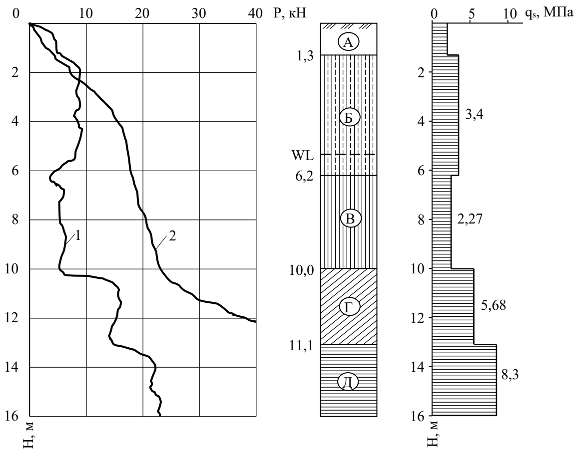
Рис. 5.16. Результати статичного зондування суглинків: а – графіки; б – геологічна колонка; в – еюра зондування; 1 – графік, побудований за результатами зондування розширеним наконечником; 2 – графік, побудований за результатами зондування конусом-зондом; А – чорнозем; Б – суглинок твердий; В – суглинок м'якопластичний; Г – суглинок тугопластичний; Д – глина тугопластична
