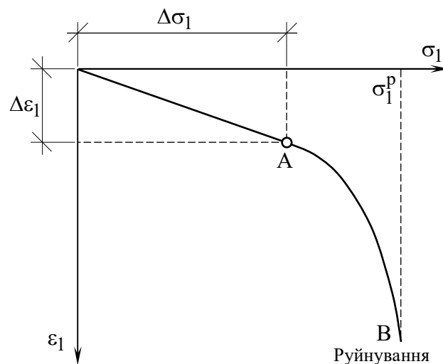
Рис. 4.9. Графік залежності відносної вертикальної деформації зразка ґрунту \varepsilon_1 від напруги \sigma_1 за результатами випробувань ґрунту в стабілометрі
