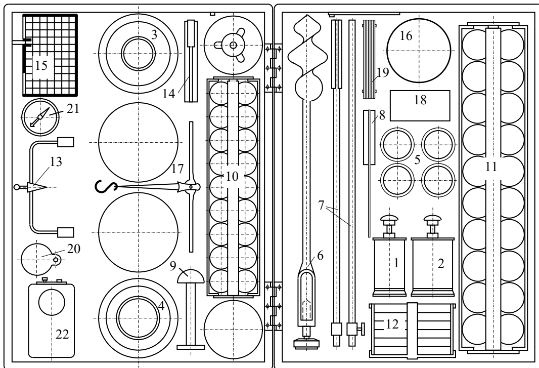
Рис. 5.10. Польова лабораторія І.М.Литвинова: 1, 2 – пристрої для відбору монолітів ґрунту; 3, 4 – опорні кільця; 5 – ґрунтовідбірні гільзи; 6 – гвинтовий анкер; 7 – важелі; 8 – ніж; 9 – виштовхувач; 10, 11 – набори бюкс; 12 – компресійні бюкси і гільзи; 13, 14 – прилади для визначення числа пластичності; 15 – пристрій для визначення кута природного укосу піску; 16 – набір сит; 17 – ваги; 18 – набір важків; 19 – метр; 20 – лупа; 21 – компас; 22 – ліхтар
