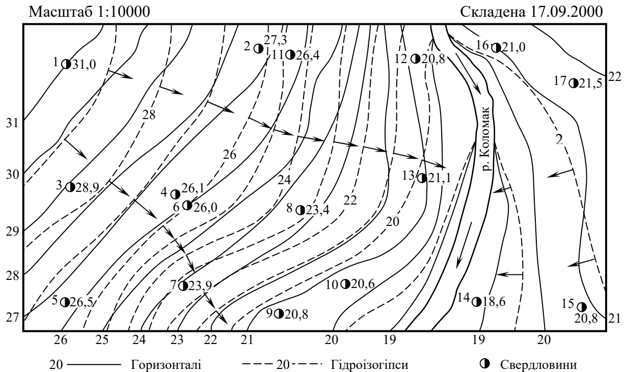
Рис. 3.21. Карта поверхні ґрунтових вод у гідроізогіпсах
