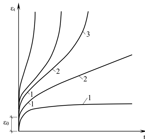
Рис. 4.22. Стадії деформацій повзучості ґрунту в часі: 1 – згасаюча; 2 – стала; 3 – прогресуюча
