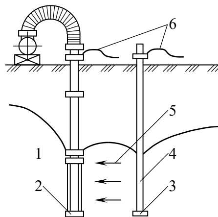
Рис. 2.20. Установка для електроосушення: 1 – голкофільтр; 2 – катод; 3 – анод; 4 – труба (стрижень); 5 – напрям переміщення води; 6 – джерело постійного струму
