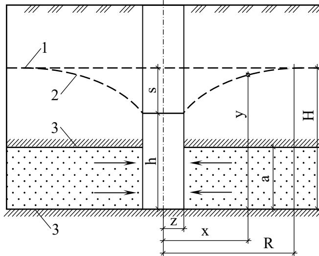
Рис. 3.13. Розрахункова схема припливу води до досконалого колодязя в напірному водоносному шарі: 1 – статичний рівень ґрунтової води; 2 – лінія депресії; 3 – водотривкий шар
