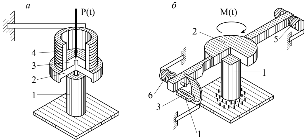
Рис. 4.26. Схема лабораторної установки для визначення власної частоти коливань зразка ґрунту: а – поздовжніх; б – крутильних
