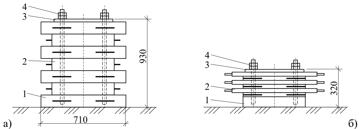
Рис. 4.25. Інвентарний штамп для визначення узагальнених пружних характеристик ґрунту: а – високий; б – низький
