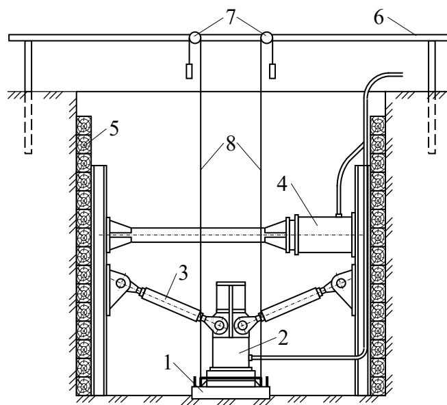
Рис. 5.11. Схема установки для випробування ґрунту штампом розпiрної конструкції у шурфі: 1 – штамп; 2 – домкрат для навантаження штампа; 3 – гвинтові упори; 4 – домкрат для горизонтального розпору; 5 – вiнцеве крiплення; 6 – реперна система; 7 – прогиномiр; 8 – дрiт
