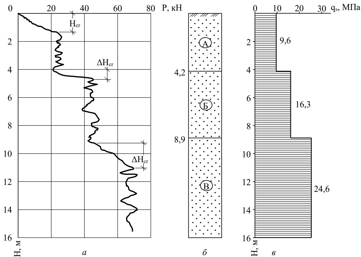
Рис. 5.17. Результати статичного зондування піску: а – графік; б – геологічна колонка; в – епюра зондування; А – пісок дрібний середньої щільності; Б – пісок середньої крупності; В – пісок середньої крупності, щільний
