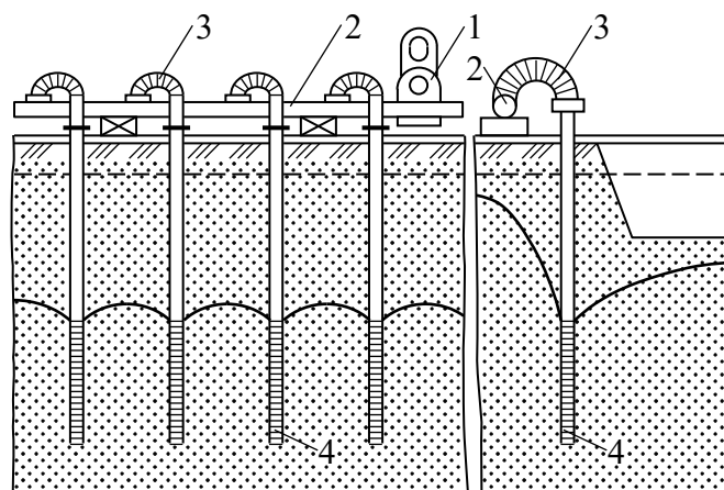
Рис. 2.19. Схема голкофільтрової установки: 1 – насосний агрегат; 2 – колекторна труба; 3 – шланг; 4 – голкофільтр
