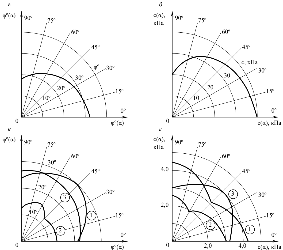
Рис. 4.20. Приклади квадрантів годографів характеристик міцності для ґрунтів з природною анізотропією за даними: а, б – професора О.В. Школи; в, з – професора М.Ю. Абелєва: 1 – лесовий суглинок у природному стані; 2 – він же у зволоженому стані; 3 – лесоподібний супісок у природному стані
