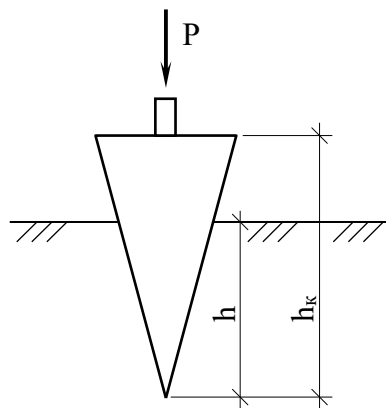
Рис. 4.14. Схема penetраційних досліджень ґрунту
