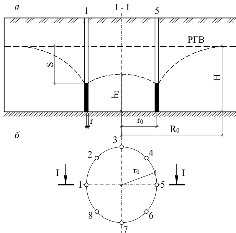
Рис. 3.16. Розрахункова схема водозниження: а – розріз по I-I; б – контур із 8 свердловин
