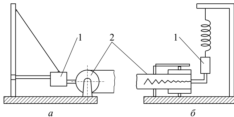
Рис. 2.5. Принципові схеми сейсмографів для реєстрації коливань: а – горизонтальних; б – вертикальних; 1 – маятник; 2 – записуючий пристрій
