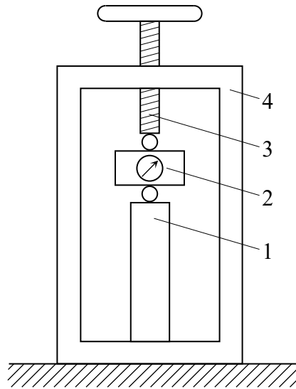
Рис. 4.24. Схема динамометричного приладу для дослідження ґрунту на релаксацію: 1 – зразок ґрунту; 2 – динамометр; 3 – гвинт домкрата; 4 – рама приладу
