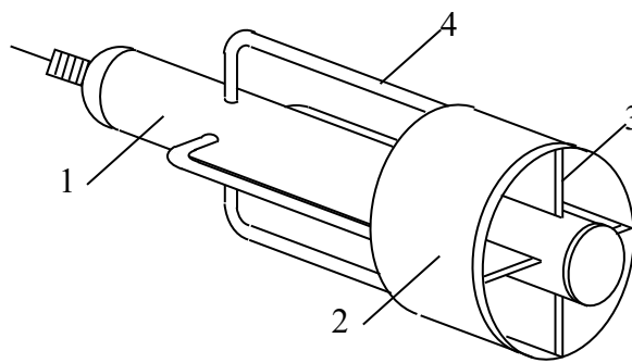
Рис. 5.1. Ударний стакан для проходження «дудок»: 1 – центральна труба; 2 – корпус; 3 – ножі; 4 – напрямна
