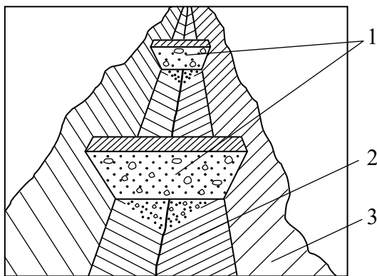
Рис. 2.12. Укріплення дна ярів за допомогою загат (гребель): 1 – кам'яні загати; 2 – дно яру; 3 – схил яру
