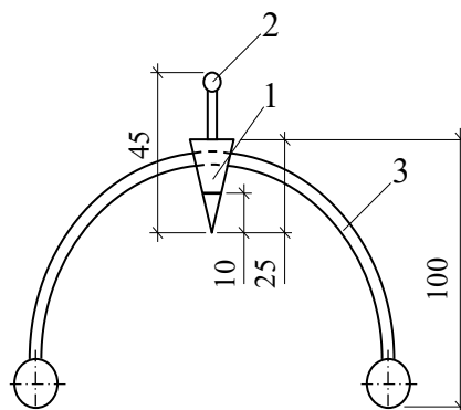
Рис. 5.18. Балансирний конус: 1 – конус; 2 – ручка; 3 – балансирний пристрій
