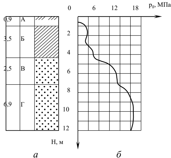
Рис. 5.15. Графік динамічного зондування: а – геологічна колонка; б – графік зондування; А – чорнозем; Б – суглинок; В, Г – піски
