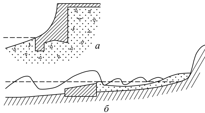
Рис. 2.18. Споруди для захисту берегів морів: a – хвилевідбійна стінка; б – підводний хвилелом
