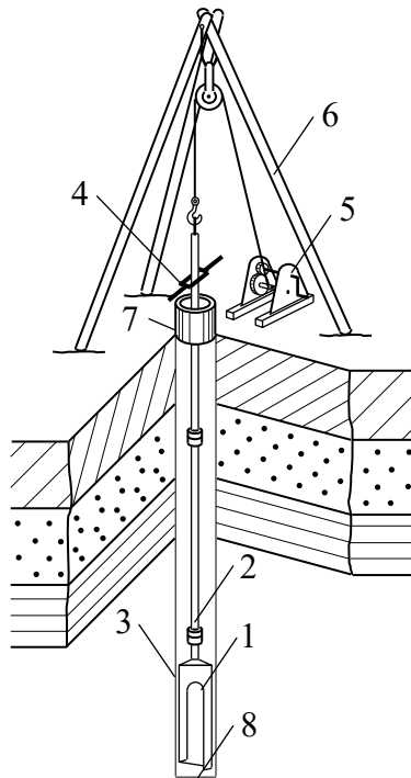
Рис. 5.3. Бурова установка для ручного ударно-обертального буріння: 1 – буровий інструмент; 2 – штанга; 3 – обсадна труба; 4 – хомут; 5 – лебідка; 6 – копер; 7 – устя свердловини; 8 – забій
