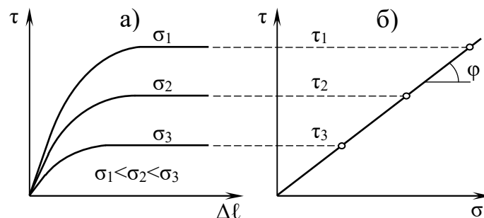
Рис. 4.11. Графіки опору зрушенню сипучого ґрунту: а – переміщень при зрушенні; б – граничного опору при зрушенні
