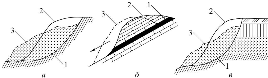
Рис. 2.33. Класифікація зсувів за Ф.П. Саваренським: а – асеквентний; б – консеквентний; в – інсеквентний; 1 – глина; 2 – схил до зсуву; 3 – схил після зсуву
