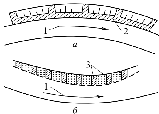
Рис. 2.13. Укріплення берегів річок: а – струменеспрямівною дамбою; б – напівзагатами; 1 – напрям течії; 2 – дамба; 3 – буни
