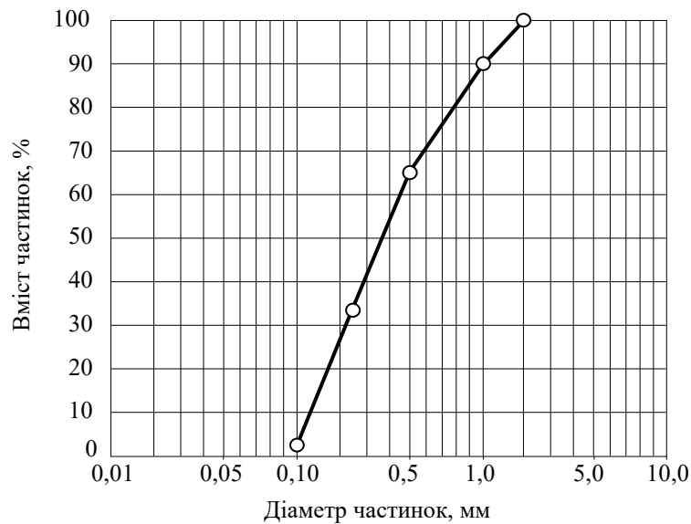
Рис. 4.2. Сумарна крива гранулометричного складу піску
