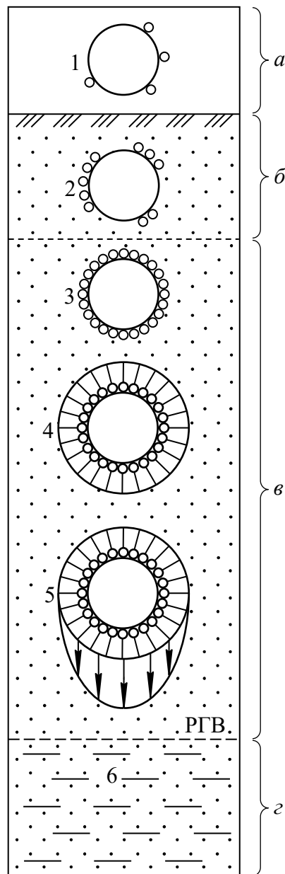
Рис. 3.2. Види води в гірських породах: a – атмосфера; б – повітряно-суха порода; в – волога порода; г – порода, насичена водою; 1, 2 – частинки з неповною гігроскопічністю; 3 – частинки з повною гігроскопічністю; 4, 5 – частинки з плівковою водою; 6 – гравітаційна вода
