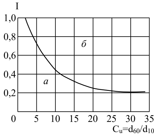
Рис. 2.22. Графік В.С. Істоміної, що показує залежність допустимих градієнтів від ступеня неоднорідності ґрунту: а – зона допустимих градієнтів; б – зона недопустимих градієнтів
