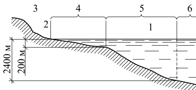
Рис. 2.16. Схема дна Світового океану: 1 – рівень моря; 2 – пляж; 3 – берегова стінка; 4 – материкова обмілина; 5 – континентальний схил; 6 – ложе Світового океану
