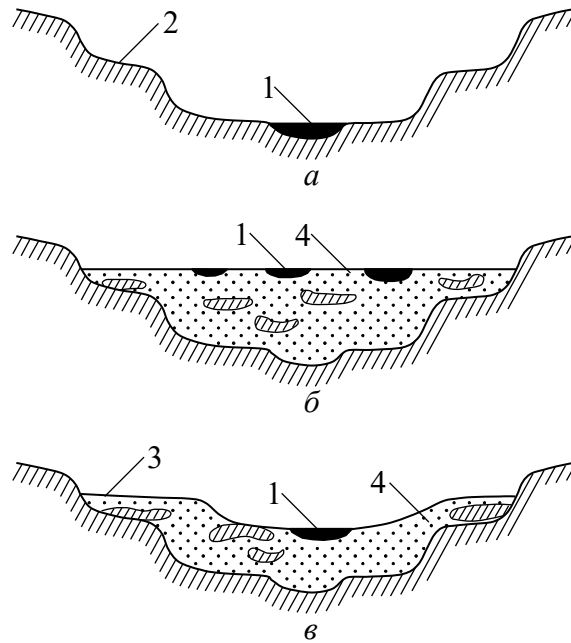
Рис. 2.10. Схема утворення річкових долин: а – ерозійної; б – акумулятивної; в – акумулятивної при зниженні базису ерозії; 1 – річка; 2 – ерозійна тераса; 3 – акумулятивна тераса; 4 – алювій
