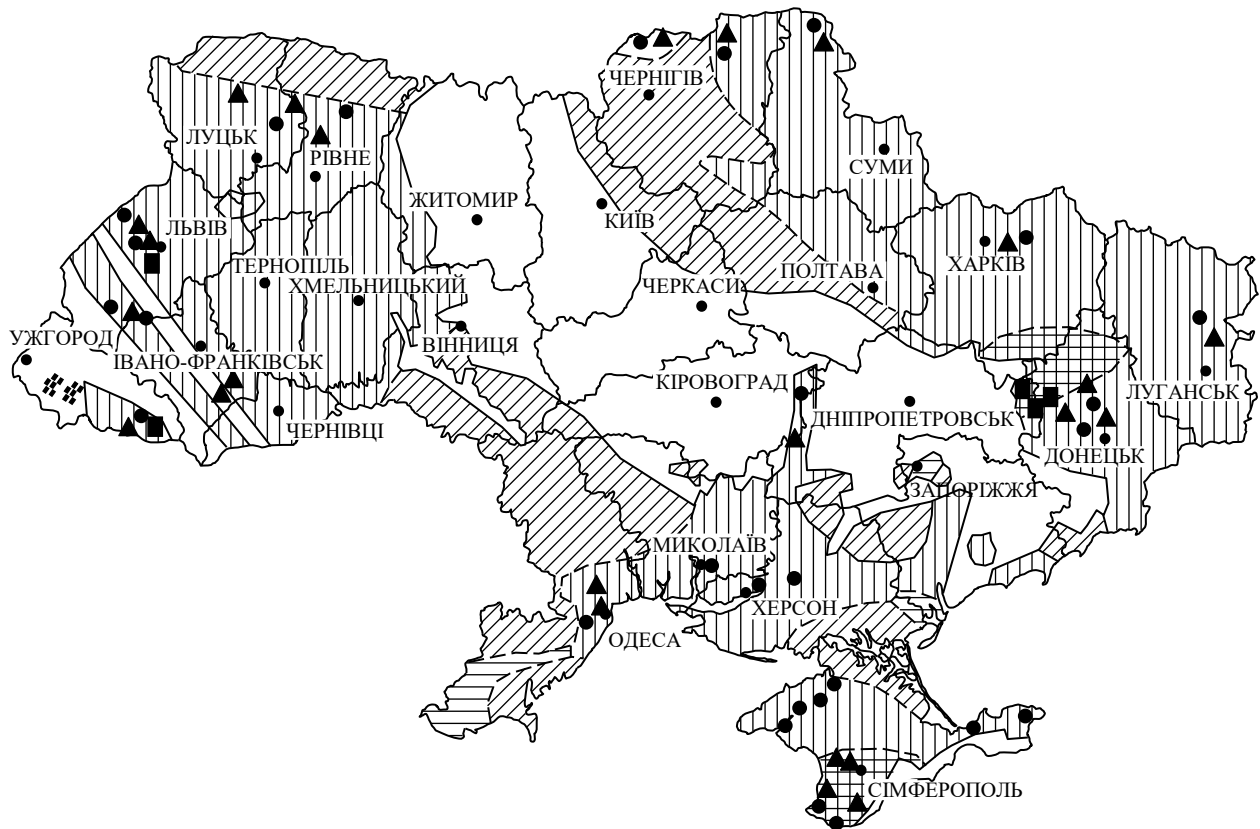
Рис. 2.29. Ступінь карстнебезпеки Україні (за Г.І. Черним)
