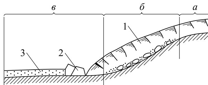
Рис. 2.14. Схематичний розріз гірського льодовика: 1 – льодовик; 2 – кінцева морена; 3 – зандрові поля; а – зона живлення; б – зона руху; в – зона розтавання
