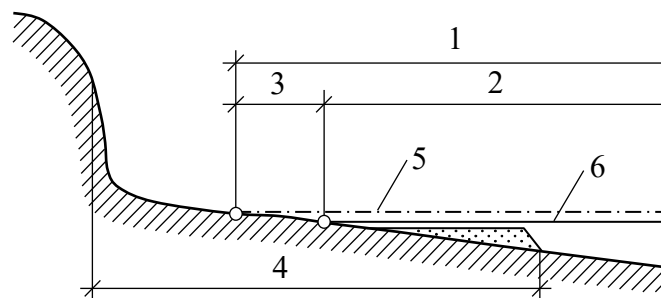
Рис. 2.17. Хвилеприбійна тераса розмивання: 1 – материкова обмілина; 2 – неритова зона; 3 – літоральна зона; 4 – хвилеприбійна тераса розмивання; 5 – приплив; 6 – відплив
