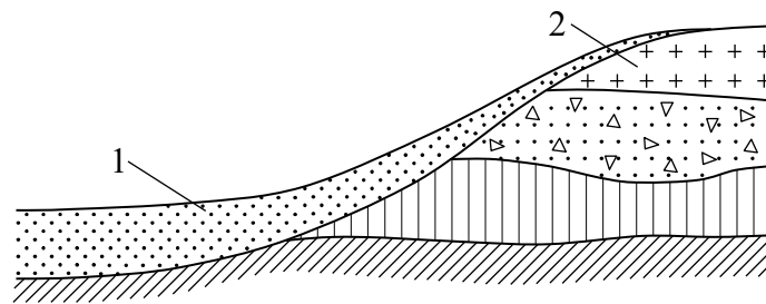
Рис. 2.7. Делювіальні відклади: 1 – делювій; 2 – корінна порода
