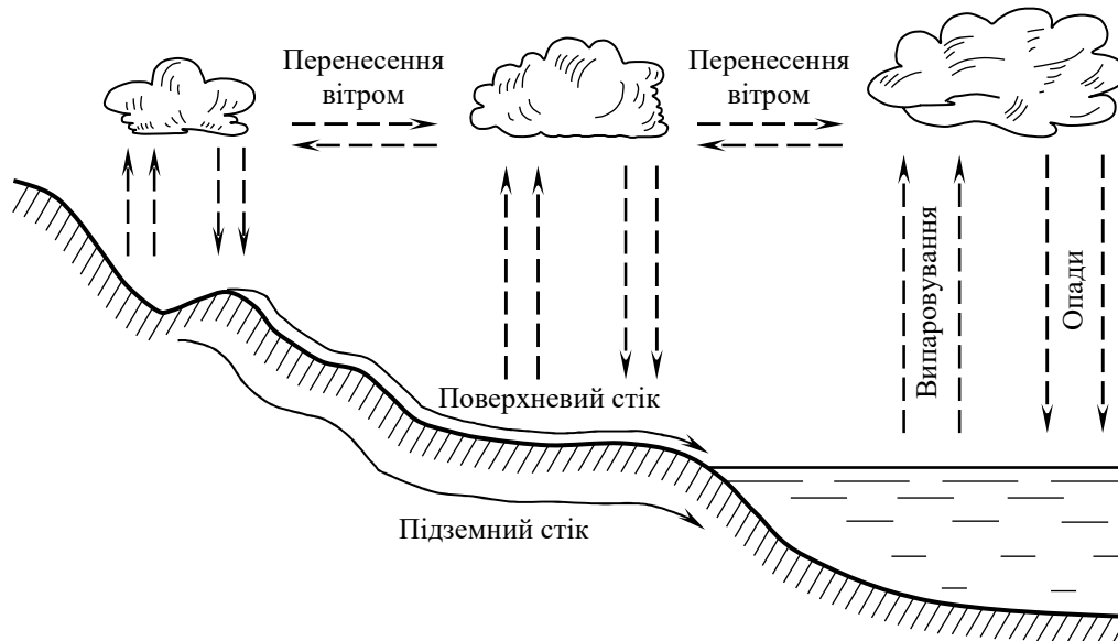
Рис. 3.1. Схема кругообігу води в природі
