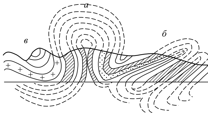
Рис. 2.1. Складки: а – антиклінальна віялоподібна; б – антиклінальна перевернута; в – синклінальна
