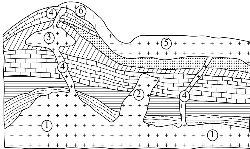
Рис. 1.3. Форми залягання магматичних гірських порід: 1 – батоліти; 2 – штоки; 3 – лаколіти; 4 – жили; 5 – покриви; 6 – потоки
