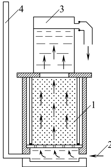
Рис. 2.21. Схема приладу В.М. Слав'янова: 1 – зразок ґрунту; 2 – подача води; 3 – прозорий циліндр; 4 – скляна трубка
