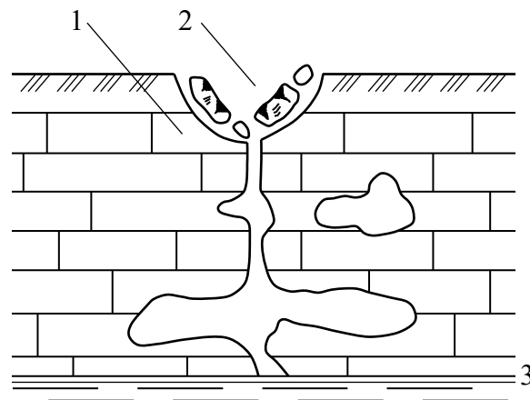
Рис. 2.27. Карстові пустоти у вапняках: 1 – вапняк; 2 – воронка; 3 – рівень карстової води
