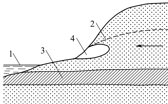
Рис. 2.23. Суфозія на схилі: 1 – рівень річкової води; 2 – рівень ґрунтової води; 3 – водотривкий пласт; 4 – ніша
