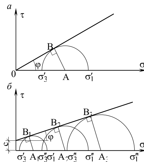
Рис. 4.13. Приклади визначення характеристик міцності ґрунтів за результатами випробувань його зразків на трьохосьове стиснення:
