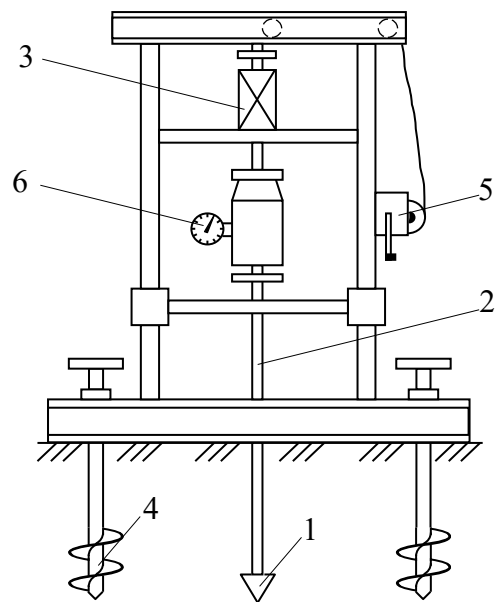
Рис. 5.14. Схема установки статичного зондування: 1 – конус; 2 – штанга; 3 – домкрат; 4 – анкер; 5 – лебідка; 6 – динамометр
