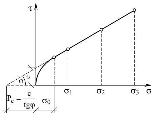
Рис. 4.12. Графік опору зрушенню зв'язного ґрунту
