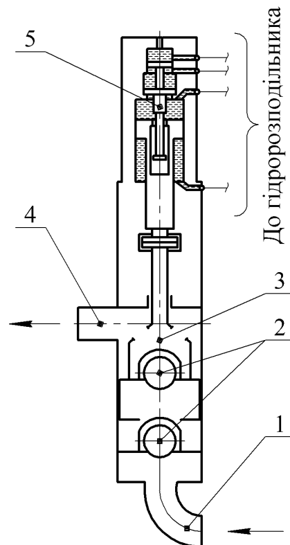
Рис. 1. Схема робочого органа розчинонасоса: 1 – усмоктувальний патрубковий; 2 – кульові клапани; 3 – проточний плунжер; 4 – нагнітальний патрубковий; 5 – золотник керування
